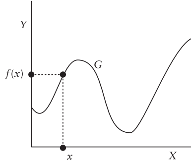
f : X \rightarrow Y fonksiyonunun grafiği
