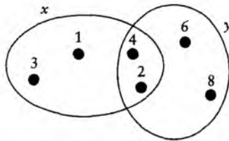
x ve y kümeleri
