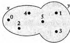
x \cup y kümesi
