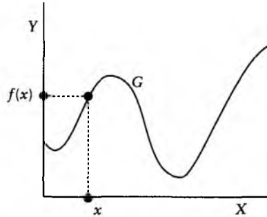
f : X \rightarrow Y fonksiyonunun grafığı
