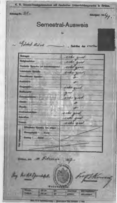
Gödel'in okul karnesi. Bütün dersler pekiyi, sadece matematik iyi...
