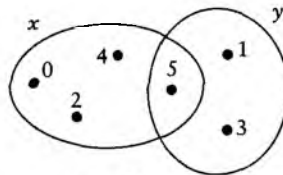
x ve y kümeleri
