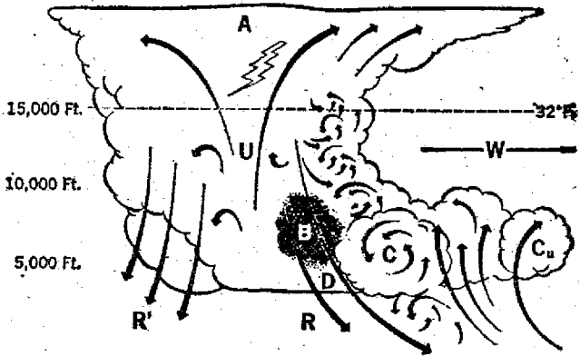
Cumulonimbus fırtına bulutunun şeması.
