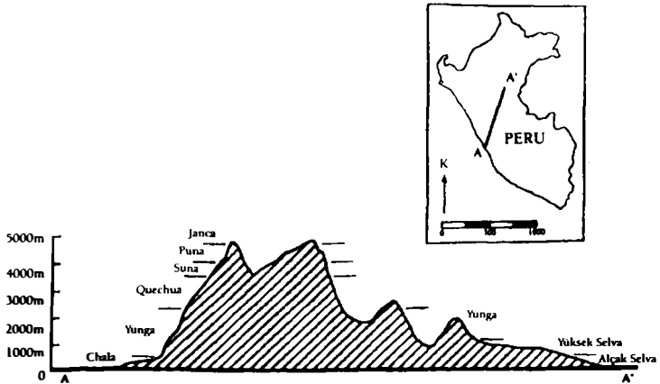
Şekil 2.10. And Dağları'nın bitki örtüsü bölgelerini ve rakımlarını gösteren enine kesiti (D'Altroy 1992).
