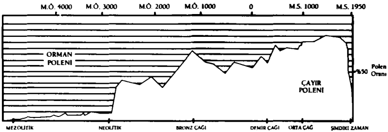
Şekil 2.2. Polen diyagramı, Thy, Danimarka (Andersen 1995).
