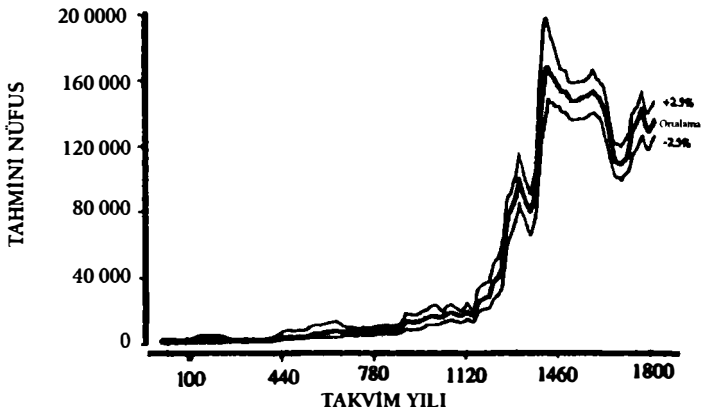
Şekil 2.9. Hawai'i Adaları için tahmini nüfus artış eğrisi (Dye ve Komori 1992).
