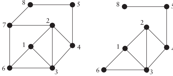
Bir çizge ve bir altçizgesi
