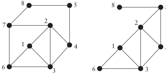
Sağdaki soldakinin bir altçizgesi değildir çünkü 2 ile 5 arasında bir kenar belirlemiştir.
