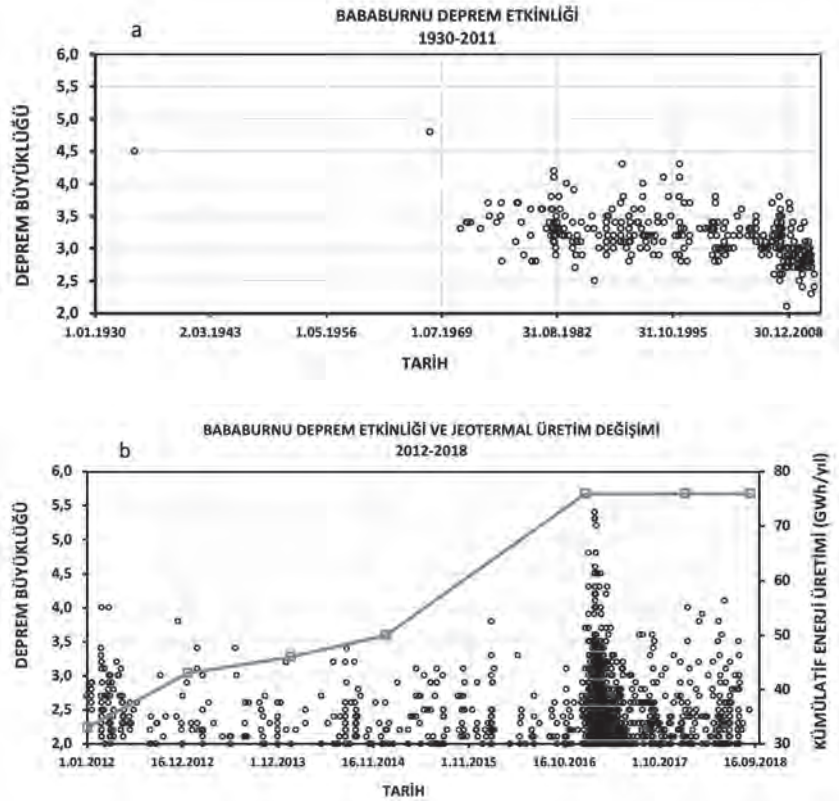
Şekil 4. Biga Yarımadası'nda Şekil 3a,b'de gösterilen alanda (a) 1930-2011 yılları ile (b) Tuzla T-1 ve T-2 jeotermal enerji üretim santrallerinin üretim yaptığı 2012-2018 yılları arasındaki deprem etkinliği grafikleri. Üstteki şekil jeotermal santralinin olmadığı 1930-2011 döneminde büyüklüğü 2.0 ve daha fazla olan depremlerin zaman içerisinde dağılımını gösterir. Altındaki şekilde ise üretimin başladığı 2012-2018 döneminde deprem oluşumu ile kümülatif jeotermal enerji üretim değeri (GWh/yıl) arasındaki ilişkiye dair grafik verilmiştir. 2012'de başlayan jeotermal üretimin özellikle küçük depremlerin sayısını artırdığı ve 2014-2017 yılları arasında jeotermal enerji üretimi artışı sonrası 2017 yılında Tuzla Fayı'nın oluşumuyla deprem fırtınasının ortaya çıkışı ilişkisi çok belirgindir.
