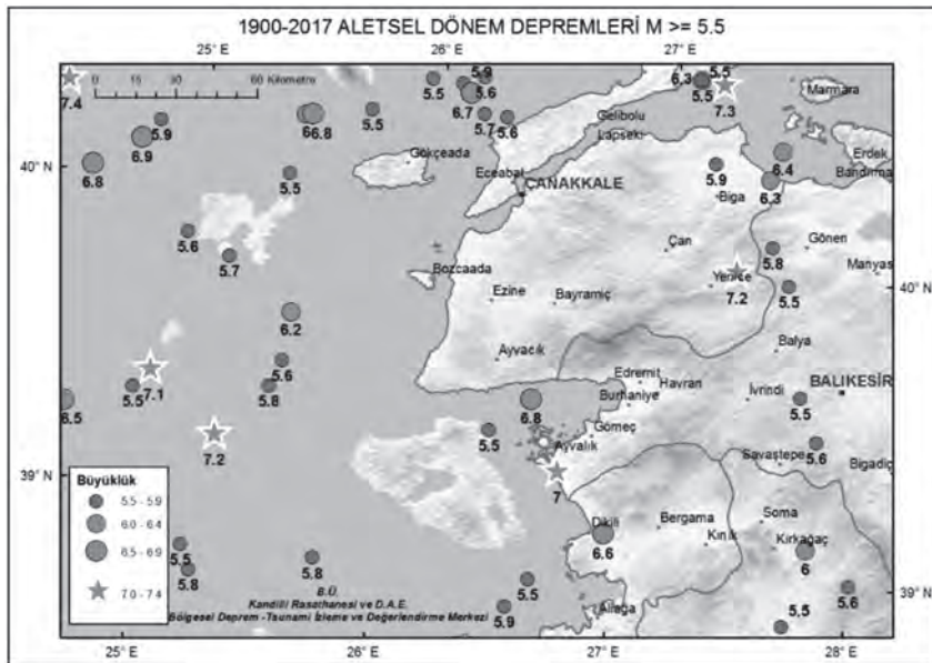
Şekil 2. Güneybatı Marmara ve kuzey Ege'de aletsel dönem (1900 yılı sonrası) hasar yapıcı önemli depremlerin konumları. Depremlerin büyüklükleri sayılarla gösterilmiştir ve ölçeklendirilmiştir. (3)
