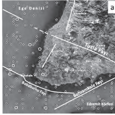
Şekil 3. Biga Yarımadası güneyindeki Bababurnu çevresinde (a) 1930-2011, (b) 2012-2018 yılları arasında büyüklüğü 3.0 ve daha fazla olan depremlerin dağılımı. Baklava semboller büyüklüğü 3.0-3.9 olan depremleri, büyük daireler büyüklüğü 4.0 ve daha fazla olan depremleri göstermektedir. T-1 ve T2 Tuzla köyündeki yıllık toplam üretim gücü 76 GWh olan santrallerin konumunu gösterir.
