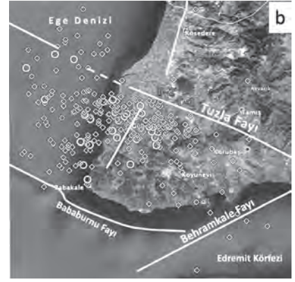
Şekil 3. Biga Yarımadası güneyindeki Bababurnu çevresinde (a) 1930-2011, (b) 2012-2018 yılları arasında büyüklüğü 3.0 ve daha fazla olan depremlerin dağılımı. Baklava semboller büyüklüğü 3.0-3.9 olan depremleri, büyük daireler büyüklüğü 4.0 ve daha fazla olan depremleri göstermektedir. T-1 ve T2 Tuzla köyündeki yıllık toplam üretim gücü 76 GWh olan santrallerin konumunu gösterir.
