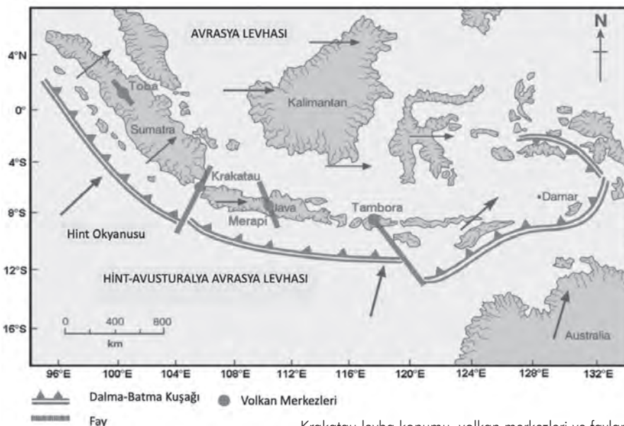
Krakatau levha konumu, volkan merkezleri ve faylar.
