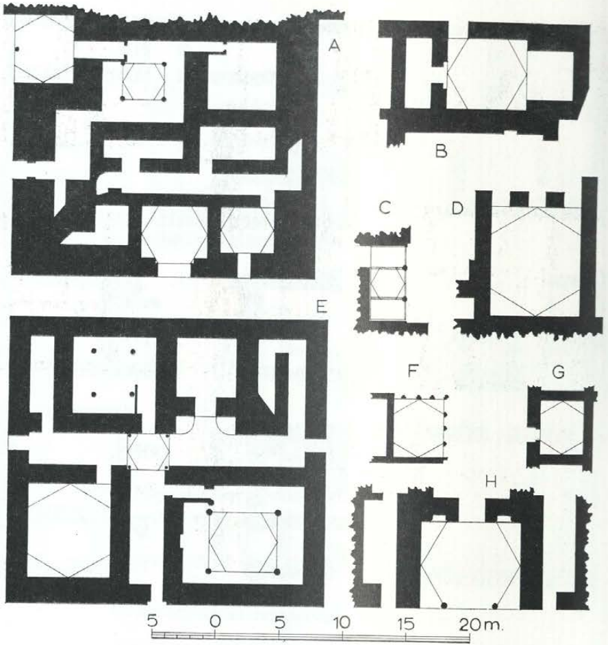
Resim 13: Erken Ortaçağ (Arap Öncesi) ve Erken İslâm Dönemi Orta Asya mimarlığında kirisli altigen tonoz örnekleri: a - Şahristan / Küçük Saray. b - Pencikent / "Obje 9" ("Sosyal amaçlı kompleks"). c - Pencikent / "Obje 9" girişin sütunlu locası. d - Varahşâ / Kızıl Salon (rekonstrüksiyon). e - Şahristan / Urtakurgan. f - Çorku / Mazar Amir Hasti Poço. g - Sayod / 19 no.lu mekân. h - Pencikent / 1 no.lu bina, plan fragmanı.
