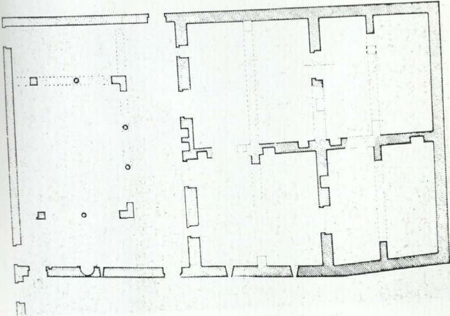
Resim 75: Karakabaklı'daki (Silifke) ev, plan.
