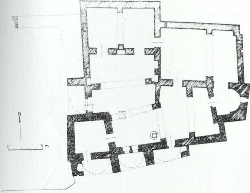
Resim 74: Sinekale'deki (Silifke) Bizans kervansarayı, plan.
