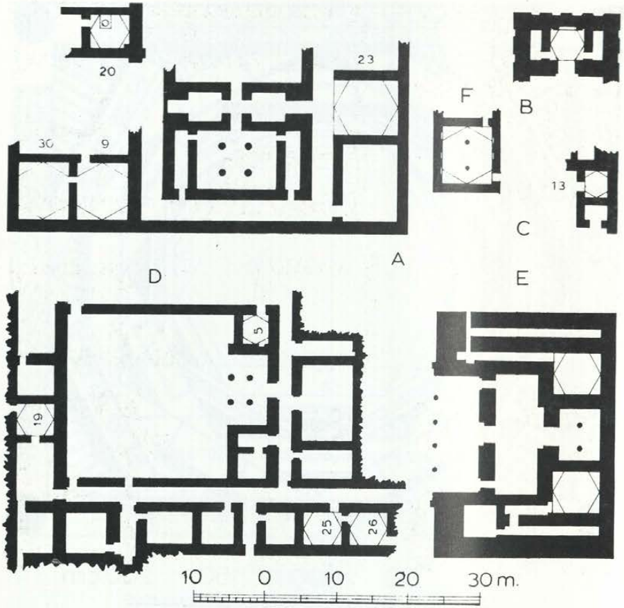
Resim 11: Orta Asya antik mimarlığında kirişli altıgen tonoz örnekleri:
