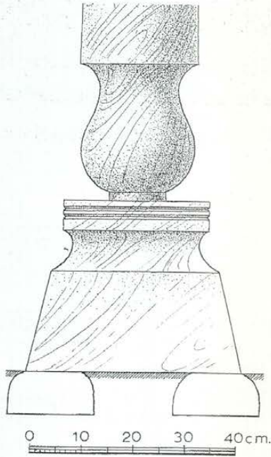
Resim 9: Urtakurgan'dan ahşap sütuna ait kaide.
