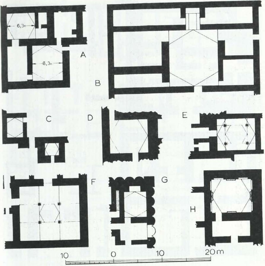
Resim 12: Erken Ortaçağ (Arap Öncesi) Orta Asya mimarlığında kirişli altıgen tonoz örnekleri:
