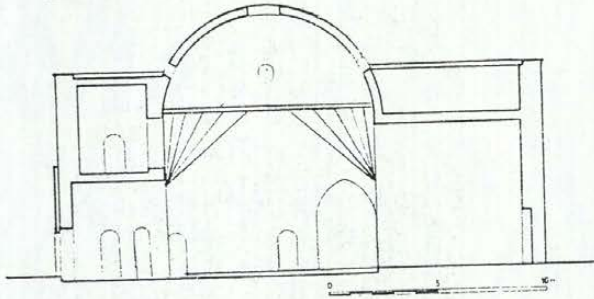
Resim 25: Karaman Ibrahim Bey İmaretı, kat planları ve kesit, (M. Sözen, Anadolu Medreseleri II).
