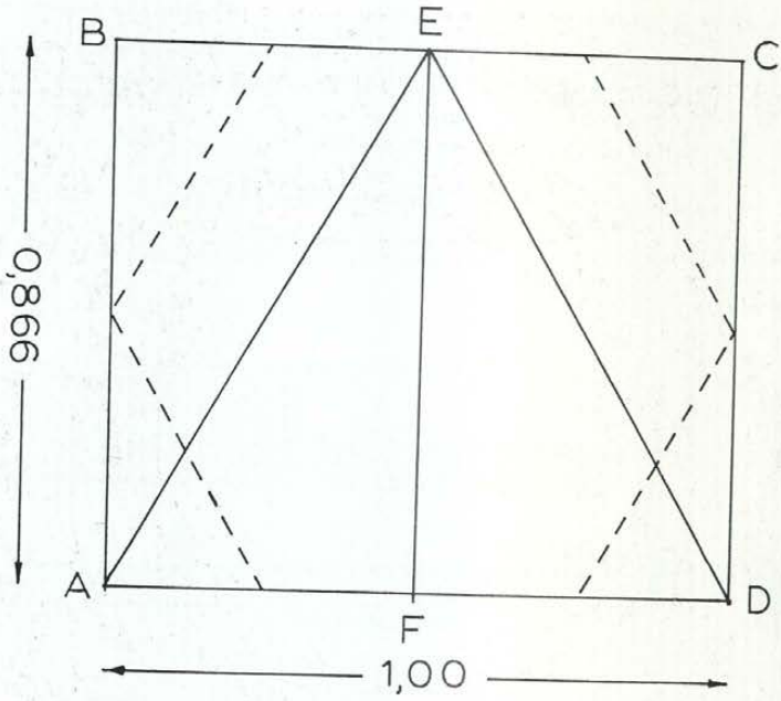
Resim 8: 1:0,866 oranındaki dikdörtgenin konstrüksiyon yöntemi.
