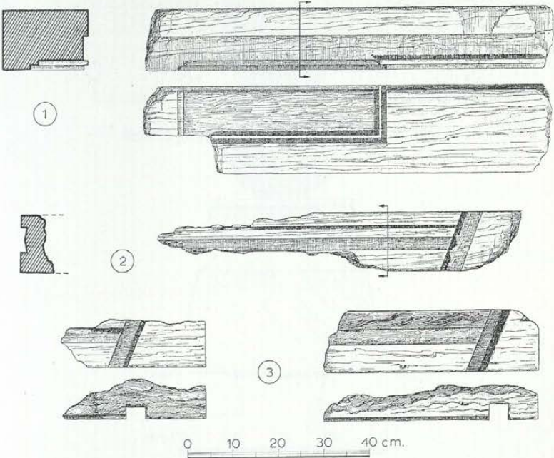
Resim 7: D, E ve F Tipi kirişler.
