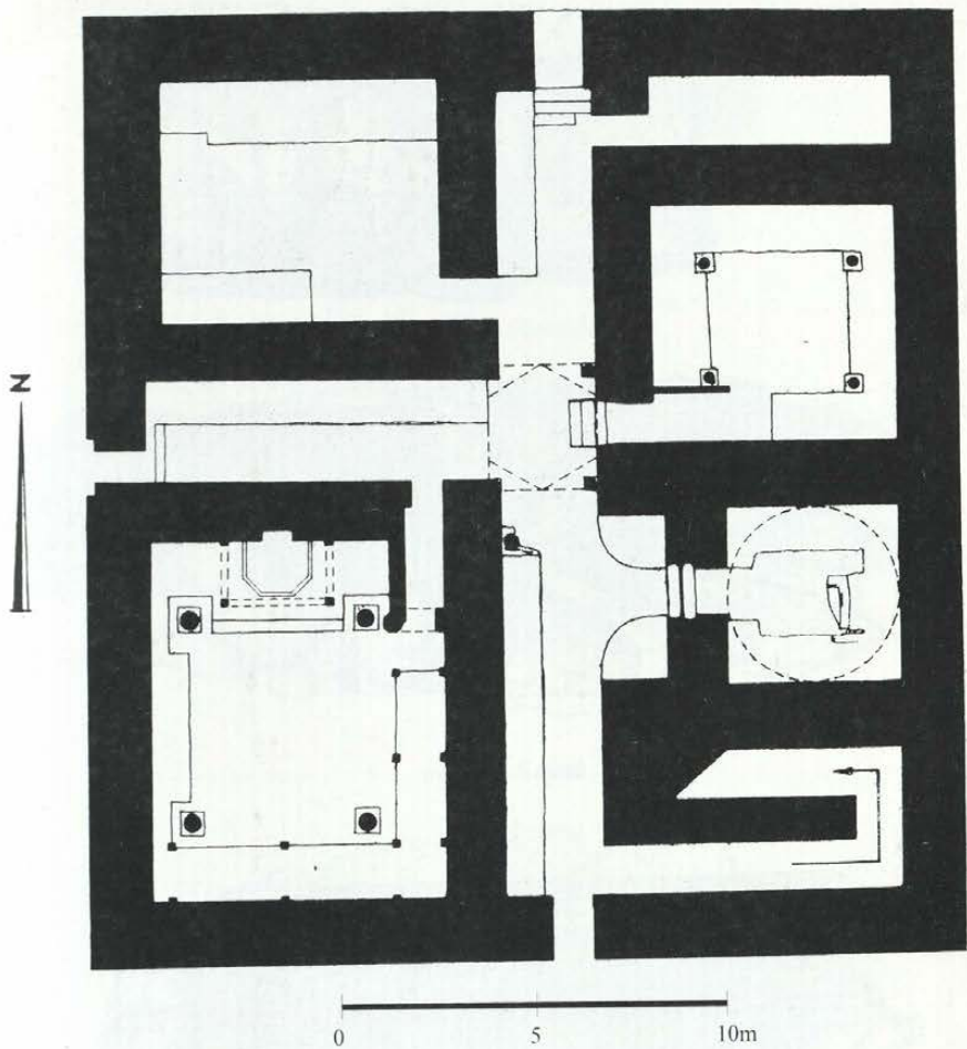
Resim 1: Urtakurgan Sarayı, Plan.
