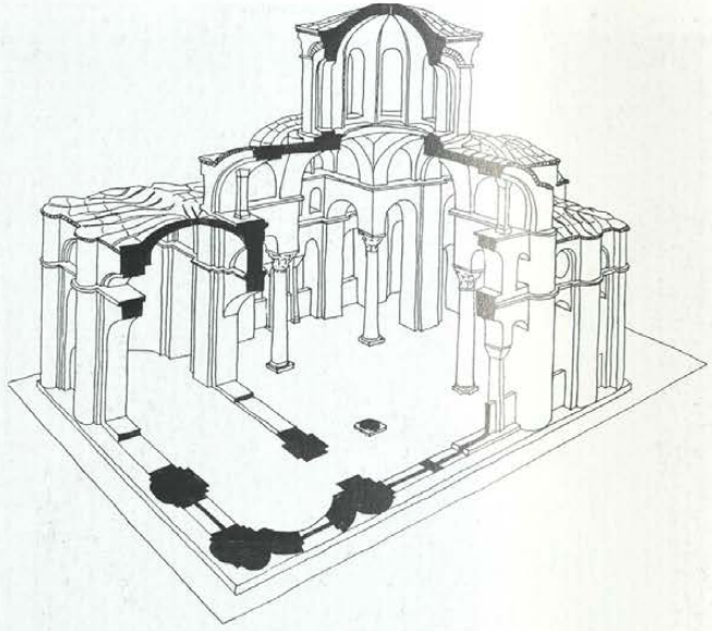
Resim 53: Myraleion (Bodrum Camii), kesit rekonstrüksiyonu, (çizim: Striker).
