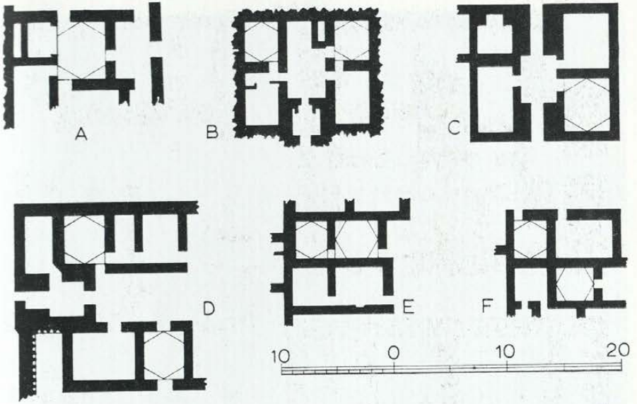
Resim 14: 10 - 13. yüzyıllar Orta Asya mimarlığından kirişli altıgen tonoz örnekleri:
