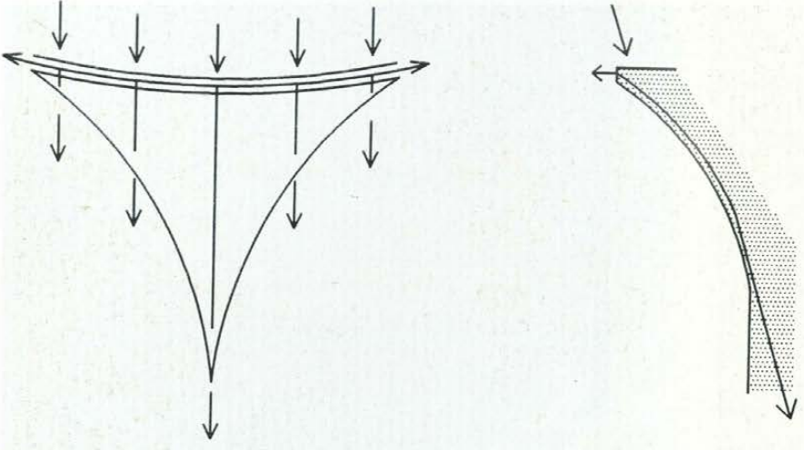
Resim 19: Pandantifte yük aktarımı, çizim.
