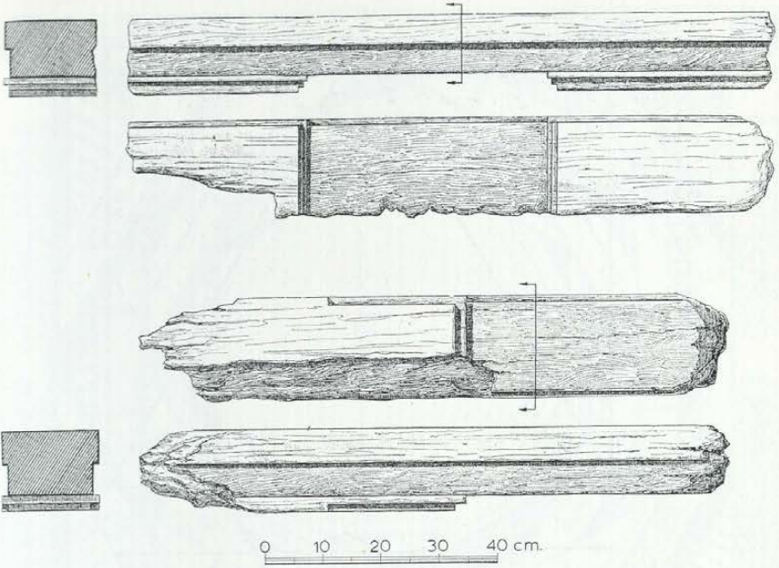
Resim 6: C Tipi kiriş.
