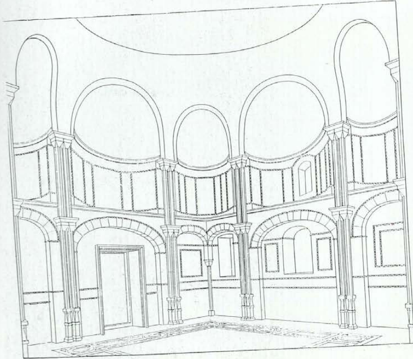
Resim 56: Nea Moni (Sakız), naosun içeriden rekonstrüksiyonu, (çizim: Orlandos).
