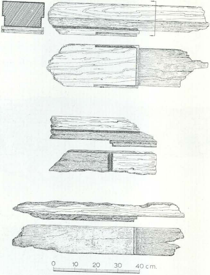
Resim 5: C Tipi kiriş.
