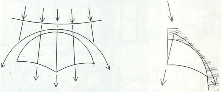
Resim 15: Trompta yük aktarımı, çizim.
