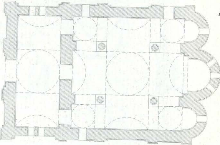
Resim 41: İdeal bir kare-içinde-haç plan, (çizim: Ş. Çorlu).
