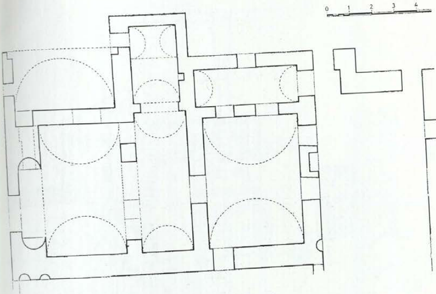
Resim 66: Side Sahil Villası, plan.
