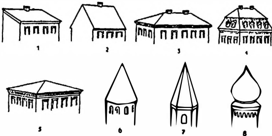
1- Sundurma çatı. 2- Beşik çatı. 3- Kırma çatı. 4- Mansard çatı. 5- Çadır çatı. 6- Konik çatı. 7- Piramit çatı. 8- Soğanbaşı çatı.
