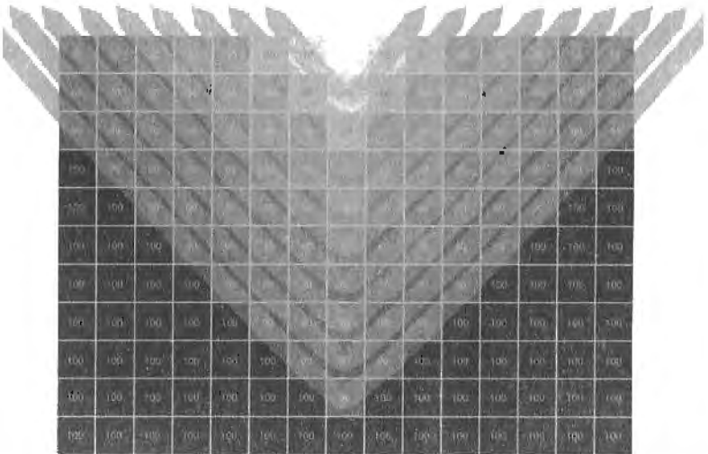
Şekil 3.8b Şekil 3.8a'daki bilgiler burada baloncuk evreninin içerisinden bakan birinin algısına göre farklı biçimde düzenlenmiştir. Aynı inflaton değerleri zaman itibarıyla aynı anlar anlamına gelmektedir. Bu nedenle çizilen eğriler aynı anı gösteren uzamsal noktalardan geçmektedir. Daha küçük inflaton değerleri zaman itibarıyla daha sonraki anları göstermektedir. Eğriler sonsuz biçimde uzayıp gidebilecektir, dolayısıyla, içeriden bakan birinin gözünde uzay uçsuz bucaksız olacaktır.
