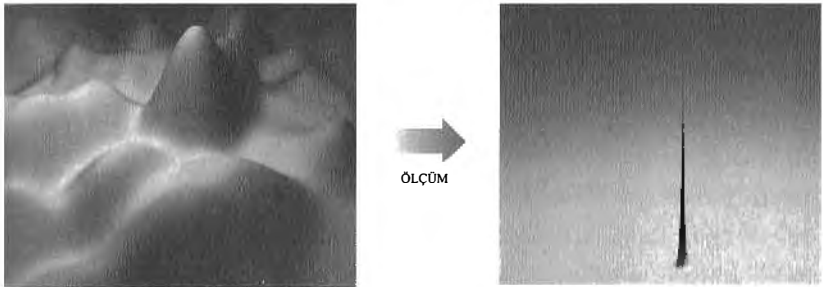
Şekil 8.6 Kuantum mekaniğinde Kopenhag yaklaşımına göre, bir parçacığın olasılık dalgası ölçüldüğünde ya da gözlemlendiğinde bir nokta hariç diğer tüm noktalarda aniden çöker. Böylece, parçacığın olası tüm konumları tek kesin bir konuma iner.
