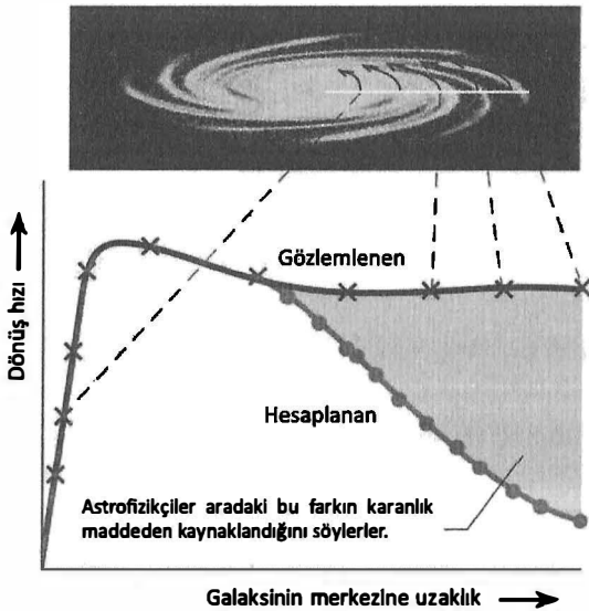
Şekil 8. Doğrudan ölçülen bir galaksinin dönüş eğrisi, parlak madde (yıldız ve gaz) dağılımından çıkarılabilecek dönüş eğrisinden farklıdır. Karanlık madde hipotezinin temelinde bu tespit vardır.
