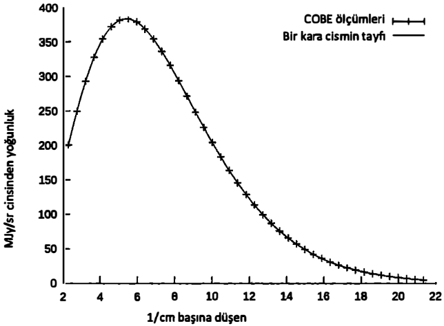
Şekil 5. 1992 yılında COBE uydusu tarafından elde edilen kozmik arkaplan ışımasının tayfı. Bu tayf tam olarak, sıcaklığı 2.725 kelvin olan bir kara cismin tayfıyla aynıdır.
