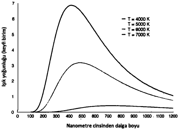
Şekil 3. Kara cismin tayfı, sadece kaynağın sıcaklığına bağlı olan bir biçime sahiptir. Sıcaklık arttığında eğrinin altında kalan alan da artar ve eğrinin maksimum noktası daha kısa dalga boylarına doğru kayar.
