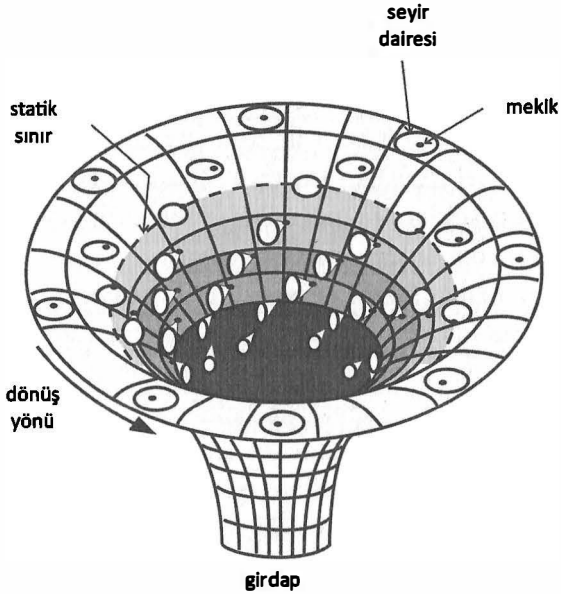
Şekil 7. Bir mekiğin döner haldeki bir kara delik etrafındaki hareketi: Seçilen yön ve hız ne olursa olsun bir an sonra kendisini seyir dairesinde bulur. (Jean-Pierre Luminet)
