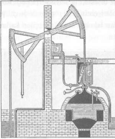
ŞEKİL 60. Newcomen'in Buhar Motoru
