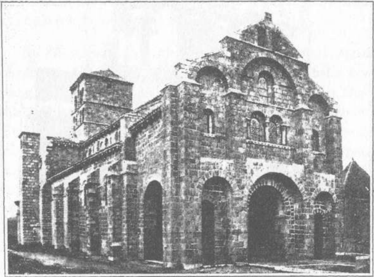
ŞEKİL 31. Fransa, Allier Bölgesindeki Châtel-Montagne Romanesk Kilisesi
