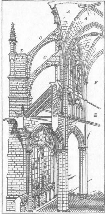
ŞEKİL 32. Amiens Katedrali'nin Enine Kesiti
