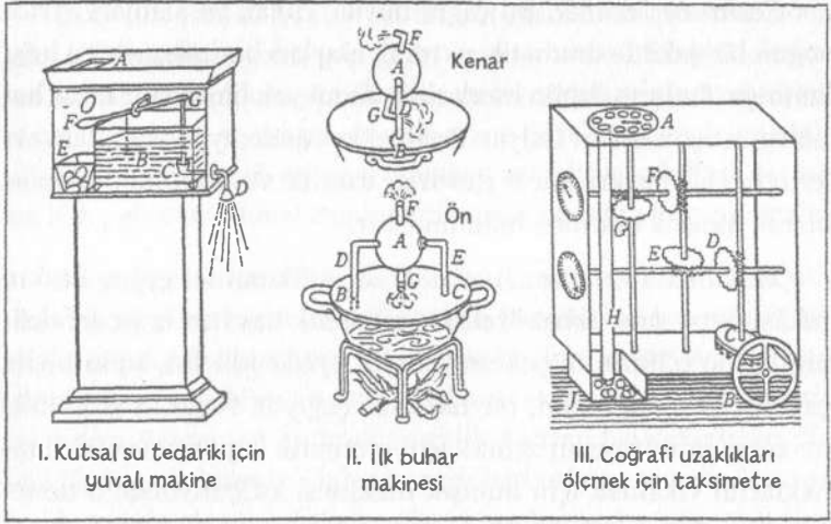
ŞEKİL 60. Hellenistik Çağ'ın Mekanik Gereçleri ve İcatları
