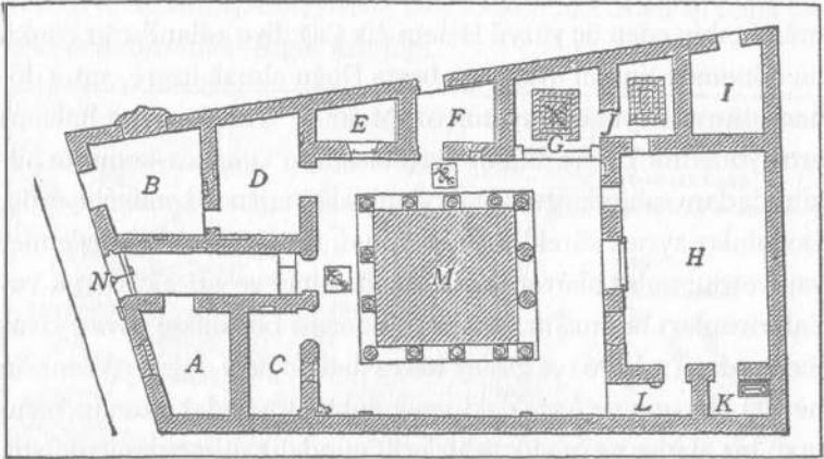
ŞEKİL 57. Helenistik Çağ'da Zengin Bir Yunanın Evinin Zemin Katı Planı
