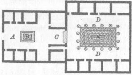
ŞEKİL 68. Sütunlu Avlusu Olan Bir Romalı Evinin Planı
