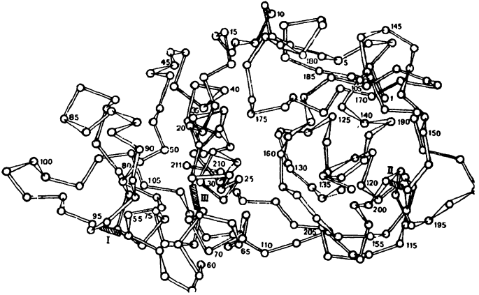
Şekil 5 Papain molekülünde peptid zincirinin katlanması- nın şematik gösterimi.
