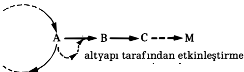
Şekil 2: Allosterik etkileşimler tarafından düzenlenen çeşitli “düzenleme tarzları”
