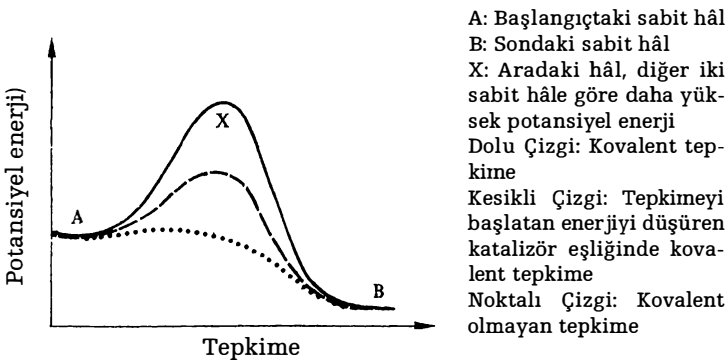
Şekil 1: Bir tepkime sırasında potansiyel enerjinin değişimini gösteren diyagram
