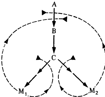
Şekil 3: Çatallı metabolik yolların allosterik düzenlenişi (Şekil 2'dekiyle aynı simgeleştirme)
