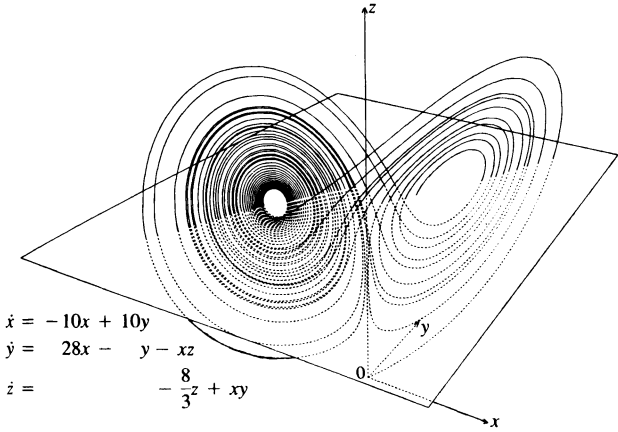
Şekil 7. Lorenz çeker. Oscar Lanford tarafından programlanan bir bilgisayar çizimi. (bkz. Lecture Notes in Math. no. 615, Sayfa 114, Berlin; Springer 1977; izni alınmış tıpkı basım)
