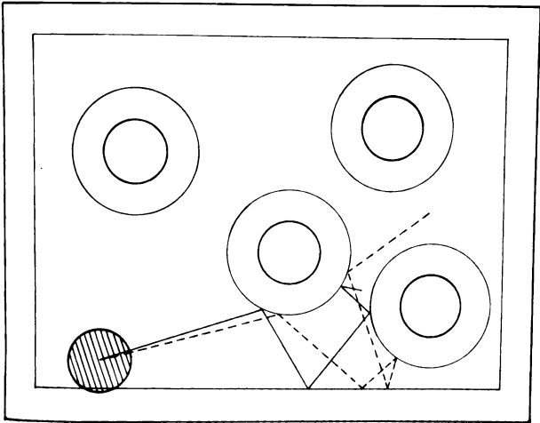
Şekil 1. Üzerinde dışbükey engeller bulunan bir bیلardo masası. Topun hareketi sol alt köşeden başlamakta olup topun merkezinin izlediği yol düz bir çizgi ile gösterilmiştir. İkinci (sanal) bir top ilkinden çok az farklı bir yönde harekete başlar (kırık çizgi). Bir kaç çarpışmadan sonra iki topun izlediği yolların birbiriyle ilgisi kalmaz.
