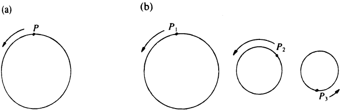
Şekil 6. (a) P ile gösterilen noktanın değişmez hızda daire biçiminde bir yörünge izlemesiyle oluşan periyodik salınım. (b) Değişik projeksiyonlarla gösterilen birden fazla mod'un üst üste gelmesi (superposition).
