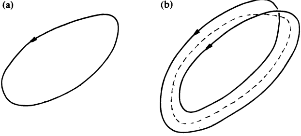
Şekil 8. Periyod katlama: (a) Periyodik bir yörünge; (b) Bunun yerini alan ve yaklaşık olarak iki kat daha uzun bir sürede tamamlanan yeni yörünge.
