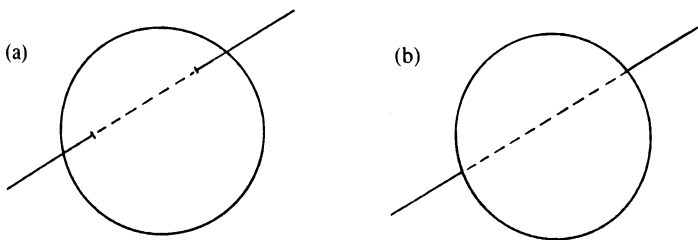
Şekil 3. (a) Bir küreyi on boyutta kesen doğru; (b) Aynı şeklin iki boyutlusu.
