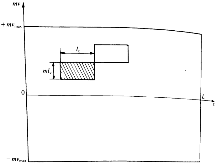
Şekil 10. Bir parçacığın evre uzayı. Büyük dikdörtgen parçacığın hareket alanıdır, küçük dikdörtgen ise kuantum belirsizliğinden kaynaklanan belirsizlik payını ölçmektedir.
