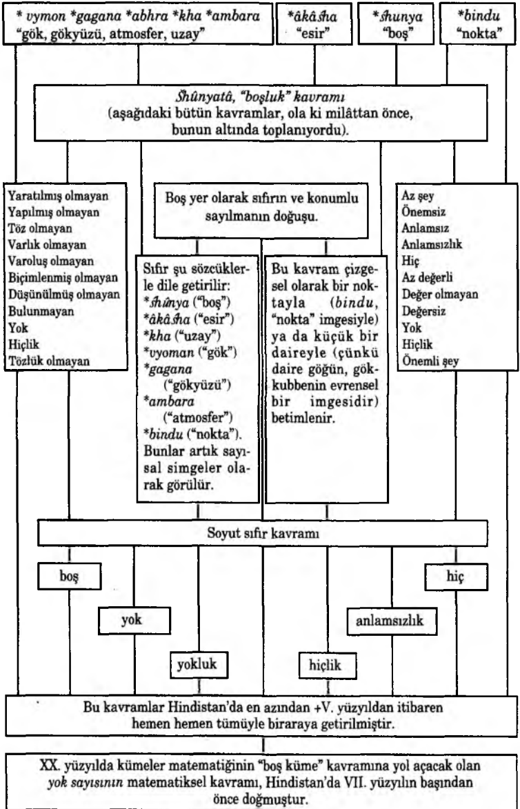
Şek. S. 11- Hint sıfırının eşsiz türdeşliği
