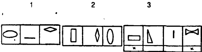
Şekil 2 - Stephenson-Spearman testi. (Problem, birinci şekilde grubunda ikinci gruptan hiçbir şeklin sahip olmadığı ortak bir özellik bulmak ve üçüncü şekil grubunda bu özelliğe sahip olan şekilleri belirtmektir. Buradaki soruda ortak özellik bir yatay eksenin varlığıdır? Bu yatay eksene sahip olan üçüncü grup şekilleri bir çarpıyla gösterilmiştir.)
