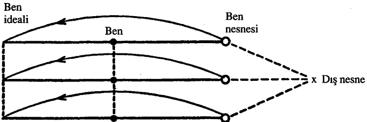
Freud'un şeması
