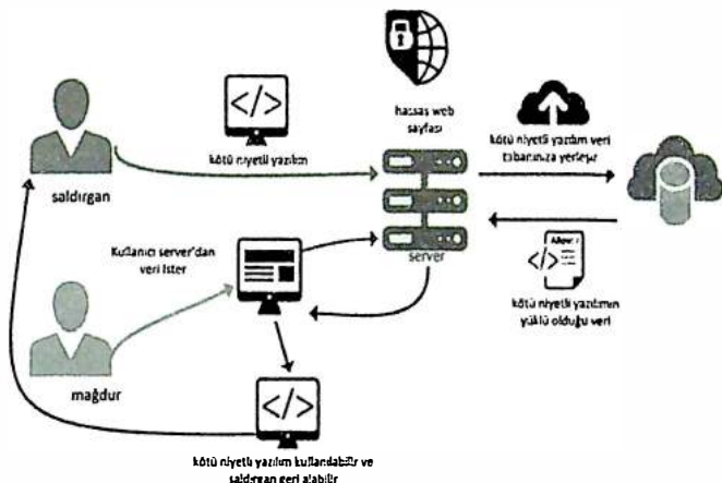
Şekil 1: Kötü amaçlı yazılım sızdırılması (drive-by attack)
