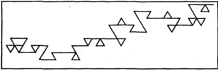
Şekil 55.1: 15. satır vectogramı
