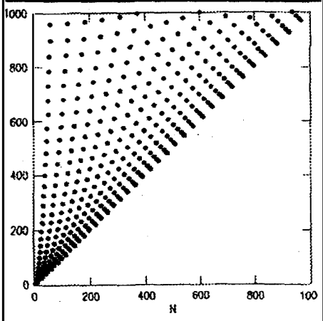
Şekil 66.1: 0 \leq n, p \leq 1,000 için çift kareseller. Bu dağılım n = p doğrusuna göre simetriktir ve alt kısmı işaretlenmemiş.
