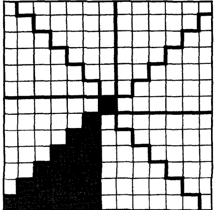
Şekil 62.1: Kare sayılar K ve Üçgen Sayılar T arasındaki derin bağ. 8T + 1 = K ifadesinin görsel bir kanıtı.
