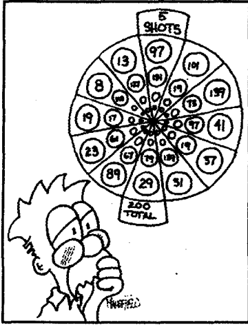
Şekil 123.1 : Zerdüş Okçuluğu Toplamları 200 eden 5 sayı var. (Çizim: Brian Mansfield)
