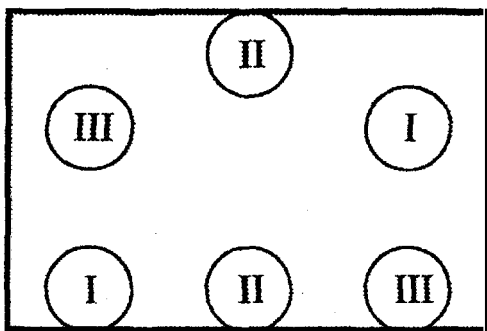
Şekil 2.1: Coliseum puzzle
