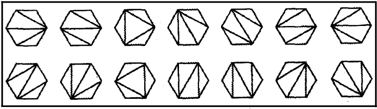
Şekil 68.1 : Bir altıgeni üçgenlere bölmek için kullanılan 14 yol.
