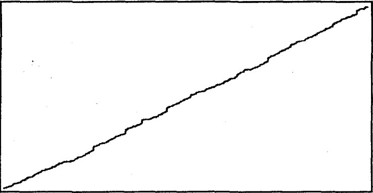
Şekil 55.3: 33. satır vectogramı
