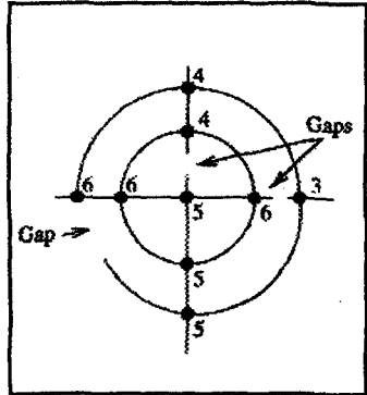
Şekil 7.2: Ağı numaralandırmak.
