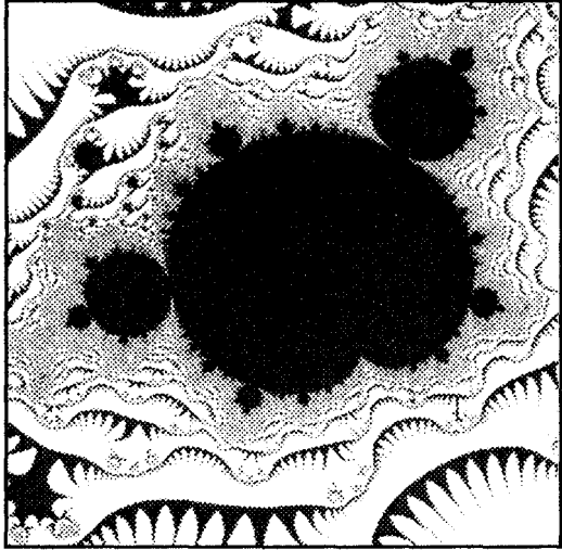
Şekil 1.2: Mandelbrot Kümesi, Guinness Rekorlar Kitabı'nda "matematikteki en karmaşık obje" olarak adlandırılmıştır. Kitapta, "Şeklin özetle matematiksel tanımı için sonsuz bilgi gerekirken istenen kalıp birkaç çizgi ile bil-
