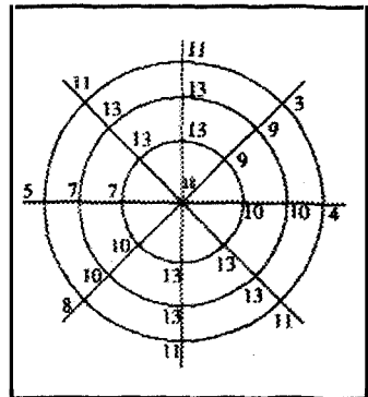
Şekil 7.3: Bir (4,3) ağı.
