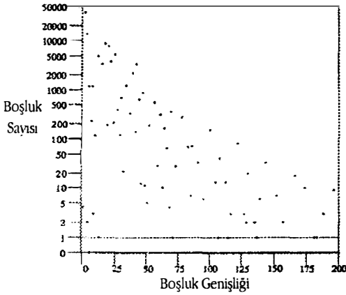
Şekil F77.1: İlk 100.000 ardışık \cup_{1,2} sayıları arasındaki ilk 100.000 boşluğun dağılımı. Her bir boşluğun olduğu zamanların sayısı, y eksenı boyunca 1 ile 50.000 arasında değerlerle ifade ediliyor. (Ken Shirriff ile işbirliği)
