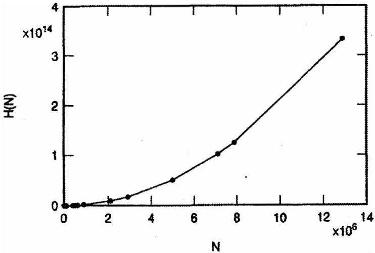
Şekil 65.2: Beşgensel sayıların dağılımı.
