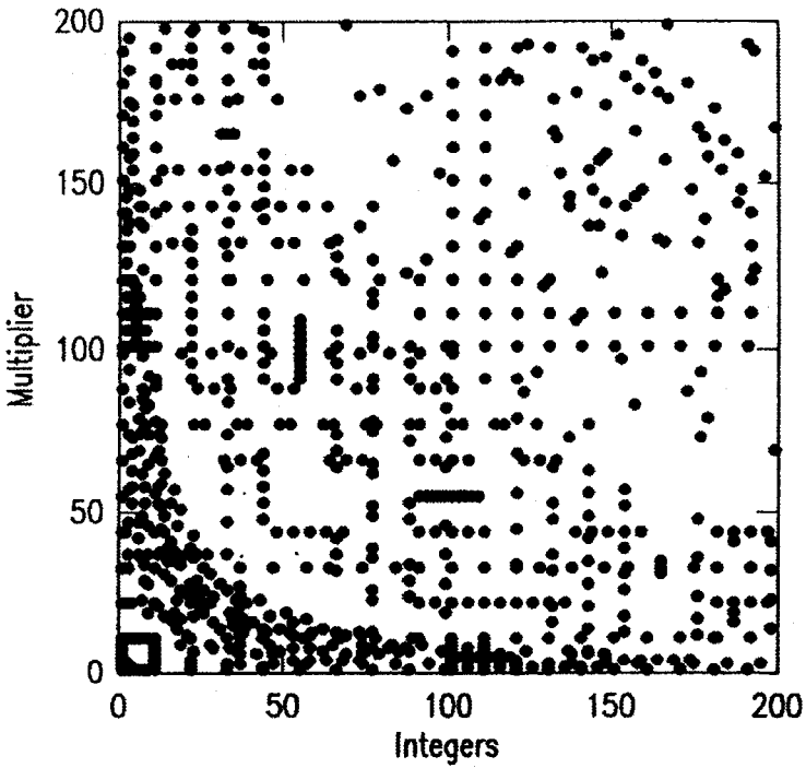
Şekil 57.1: Palindrome dağılımı. Yatay eksen x tamsayılarını, dikey eksen ise integral çarpan a 'yı veriyor. Grafikteki noktalar ise a ( x 'in Palindrome olduğunu gösteriyor).
