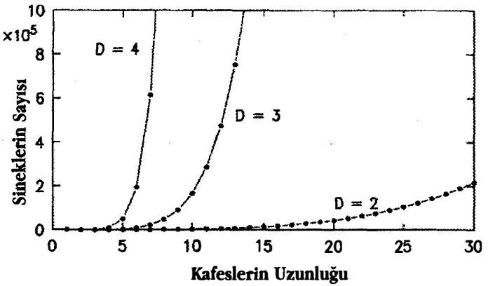
Şekil F61.2: n ölçüsünde 2, 3 ve 4 boyutlu kafeslerin ihtiva edebilecekleri sineklerin sayıları. [Dikey: Sinek Sayısı, Yatay: Kafes Ölçüsü]
