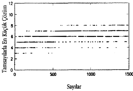
Şekil 78.1: Minimal tamsayı çözümleri. \mathcal{Q}(n) çözümleri ilk 1.500 sayı içindir. Tamsayıların sıralamaları dahil edilmemiştir.
