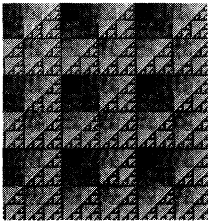
Şekil 70.1: Parçaların kalıbı. Kalıp c_{ij} = i \text{ VE-} YAj ; ( 1 < i < 800 ) ve ( 1 < j < 800 ) ile oluşturuluyor. 255 modundaki c değerleri gri gölgelerle gösteriliyor.
