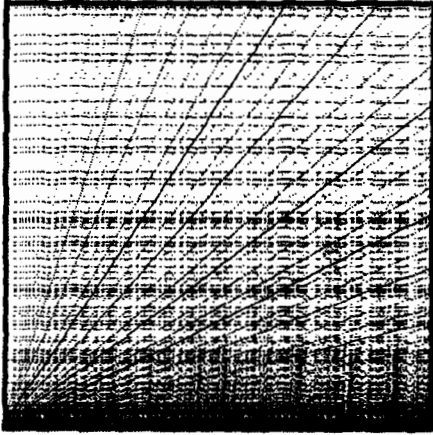
Şekil 49.2: x apsisinde 1 ile 1000 arasındaki tüm başlangıç sayılarıyla oluşan Dolu Tanesi Dizileri. Dolu Tanesi Sayılarının çizdikleri yollar, y ordinatında görülmüştür.
