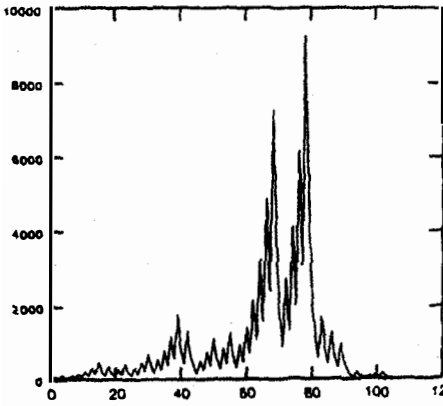
Şekil 49.1: Tek bir başlangıç sayısı, 54 ile oluşan dolu tanesi dizisi.
