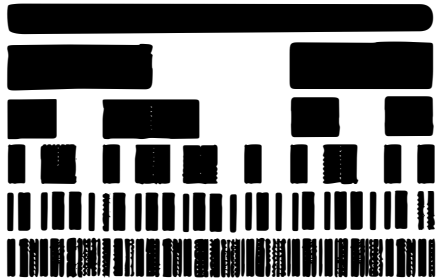
Şekil 69.1: Anaiyotik Ana Bölmeleri. A harfi koyu parçalarla, n ise beyaz boşluklarla gösteriliyor.
