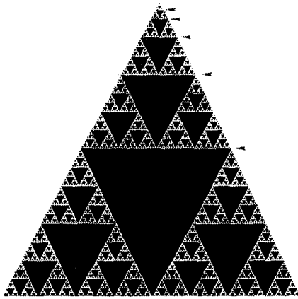
Şekil 54.1: Mod 2'de Pascal Üçgeni. Oklar her bir k m satırında bulunan merkez üçgenlerdeki ölçü değişimini gösteriyor ( m = 0, 1, 2, 3, \dots ). Burada k mod indeksi. Ölçü değişim ilişkisi tüm üçgenler için mod p 'de geçerlidir, p asal bir sayıdır. Görünen oklar 23, 24, 25, 26 ve 27.
