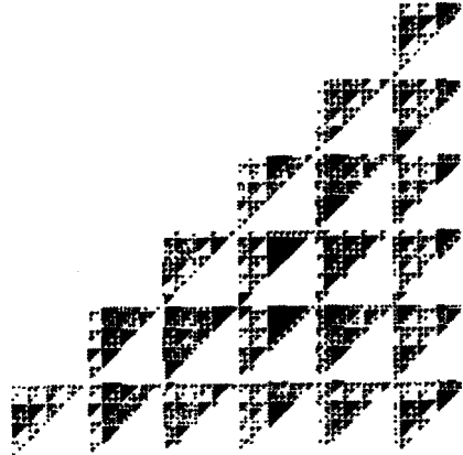
Şekil 54.4 "Pascal'ın Hayvanları" Mod 2'de Pascal Üçgeni
