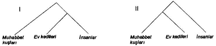
Şekil 9.6 İki karşıt kladogram. Her biri geçmiş hakkında farklı bir hipotezi temsil ediyor.
