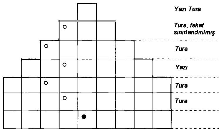
Şekil 8.1 Sınırlanmış bir stokastik süreç
