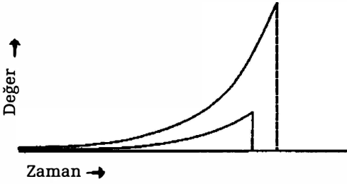
Şekil 7.2 Farklı zamanlarda mümkün olan, farklı büyüklükteki iki ödülün geleneksel (üstel) eğrileri. Özenin önceki ve sonraki ödülleri değerlendirebileceği her noktada bunların değerleri nesnel büyüklükleriyle orantılı olarak kalacaktır. (Ainslie, 2001, Breakdown of Will , s. 32.)
