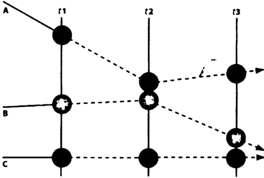
Şekil 2.3. Laplace'ın evreninin anlık görüntüsü.
