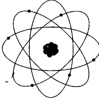
Şekil 2.1 Bohr Atom Modeli
