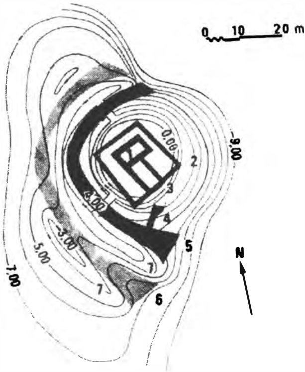
Şekil 2: Saint-Martin-de-la-Brasque (Vaucluse). Şato: onarımlarla birlik- te genel plan. Eğri aralığı: 1 m (kazı öncesi röleve). 1: kule? 2: çevre duva- rı. 3: ev. 4: giriş. 5: iç hendek. 6: dış hendek. 7: sur.
