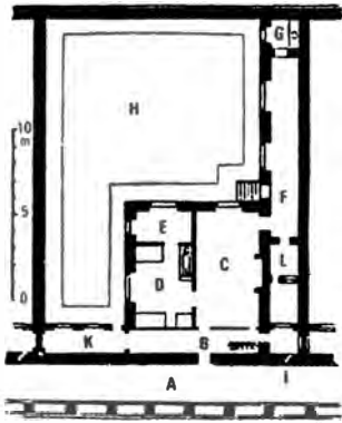
Şekil 13: Viollet-le-Duc'e göre tipik bir Chartreuse evi planı. A: arkatlı avlu galerisi, B: ilk koridor, C: ısıtılan birinci salon, D: yatak ve üç mobilya içeren hücre, E: dua bölmesi, F: üstü kapalı gezinti yeri ve sonunda tuvalet (G), H: küçük bahçe, I: besinlerin konduğu kule, K: başrahibin bahçenin içini görmesine ve keşiflere odun ve diğer ihtiyaç maddelerinin ulaştırılmasına imkân sağlayan küçük portik, L: bu maddelerin konduğu yer.
