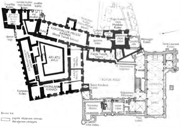
Şekil 11: Avignon Papalık sarayı. V. Urbanus'un papalığının sonunda, 1370'teki plan. Zemin kat (S. Gagnière).
