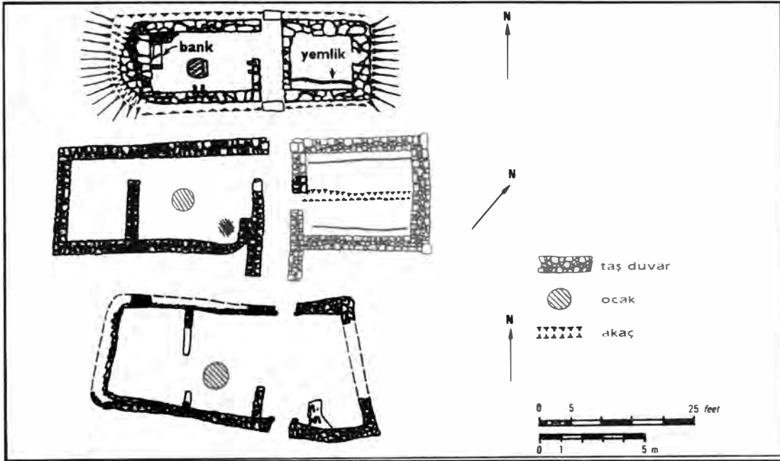
Şekil 8: Ortaçağ İngilteresi'nde, Devon ve Cornwall'da "uzun ev" planları. Bazen iki, bazen üç oda. Henüz gerçek anlamda şömine olmadığından, ortada ocaklar (M. Beresford ve J. Hurst).
