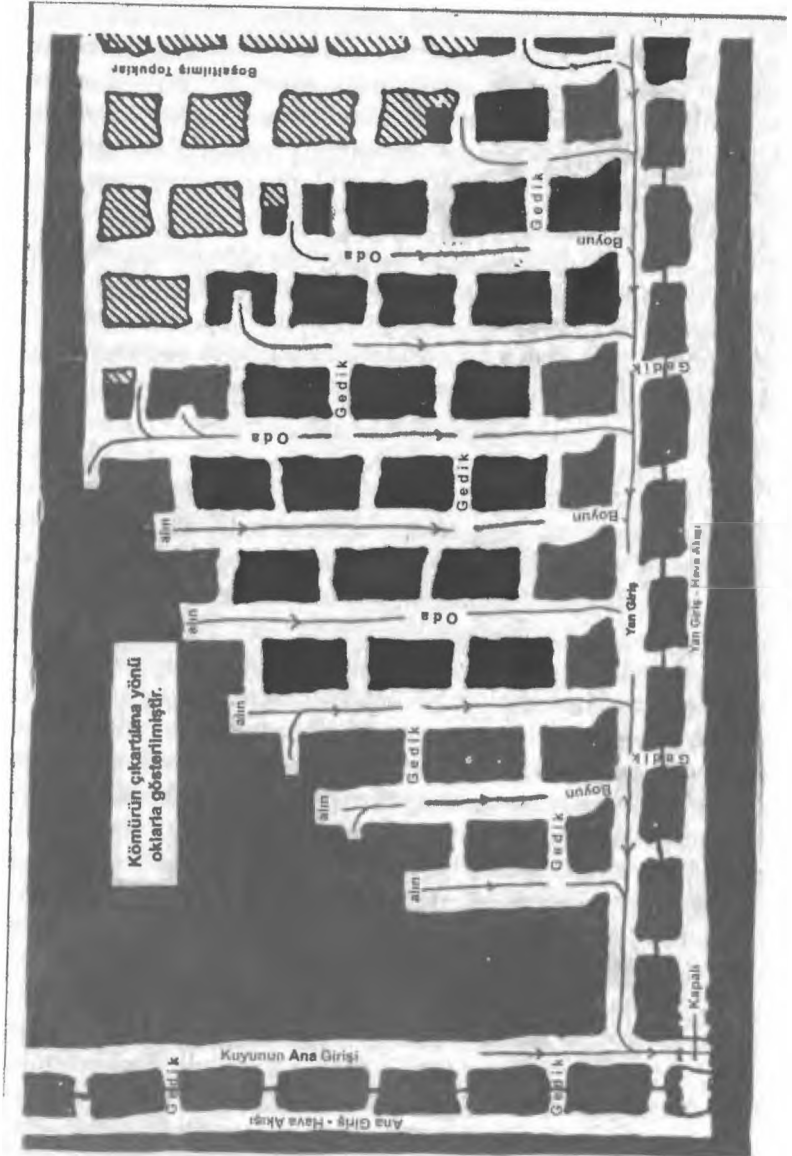
Resim 4.1 Oda-Topuk Madencilik Metodu. Kaynak: Kelth Dlx (1977), s. 5.
