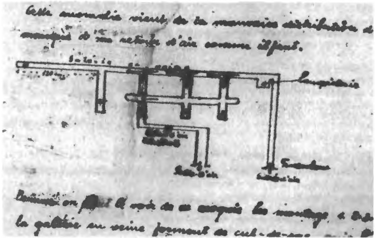
Resim 8.1 364 no'lu Alacaagzı madeni için havalandırma önerileri, Haziran 1913. Kaynak: ED 16, 76.
