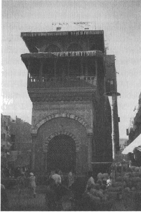
Resim 5.3 Kazdağlı Abdurrahman Kethüda'nın Kahire'nin Beynü'l-Kasreyn'indeki sebil-küttabı (1744).
