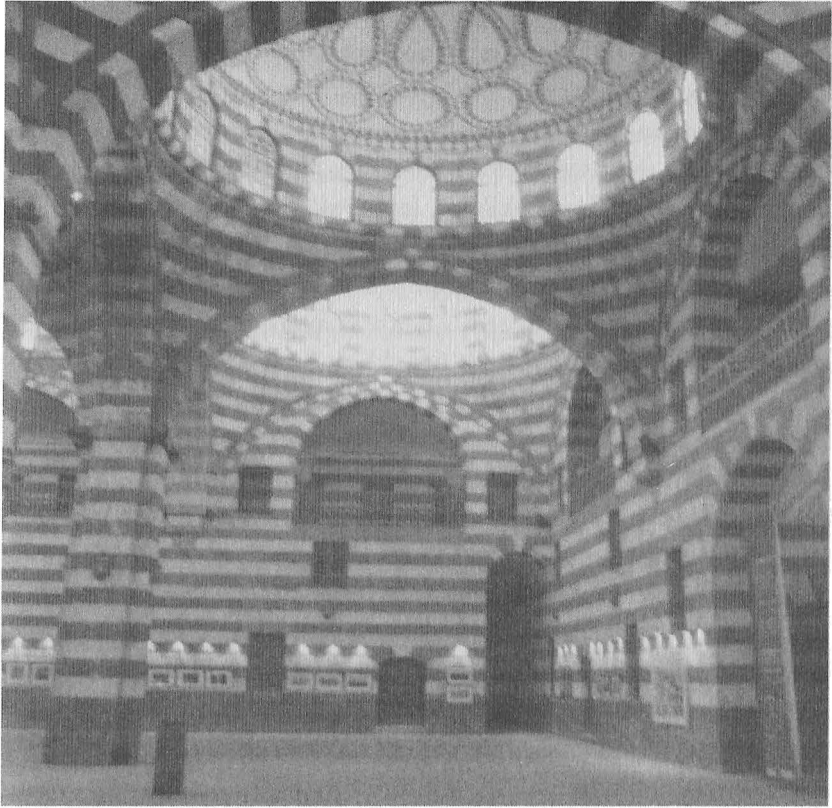
Resim 7.1 Şam'da Esad Paşa Hanı (1752). Han, 1980'lerde restore edildi ve bugün bir sergi mekânıdır. Yukarıdaki fotoğrafta bir resim sergisi görülüyor.
