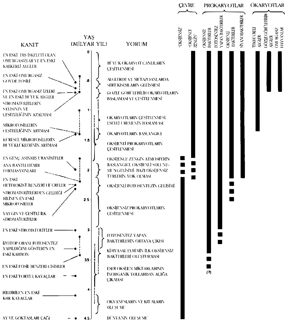
Şekil 12. Kambriyen-öncesi evrimdeki ana olaylar, fosil kayıtlarında, inorganik jeolojiden ve günümüz canlılarının metabolizma ve biyokimyası üzerine yapılan kıyaslamalı çalışmalardan gelen kanıtlar üzerine temelendirilmiş bir kronolojik sıra halinde sunulmuştur. Sonuçlar tartışmaya açıksa da, yaşam üç milyar yıl kadar önce başlamıştır (dünyanın yaşı bir milyardan biraz daha fazlayken); oksijençe zengin bir atmosfere geçiş kabaca iki milyar yıl önce gerçekleşmiştir; ökaryotlar ise 1,5 milyar yıl önce ortaya çıkmıştır.
