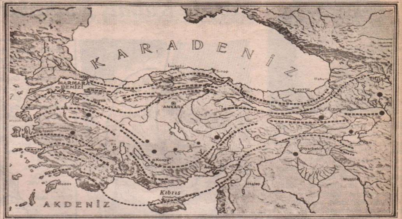
Şekil: 335. — En mühim tektonik hatlar: ● Eski Volkanlar
