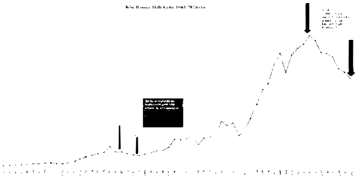
Şekil 9: Kişi Başına Millî Gelir 1961-2020
