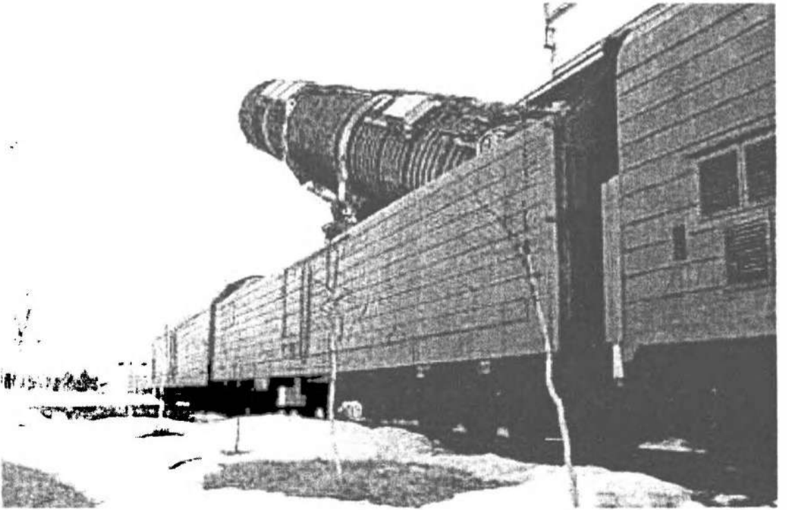
Sovyet RS-22 balistik füzesi (nükleer Katar)
