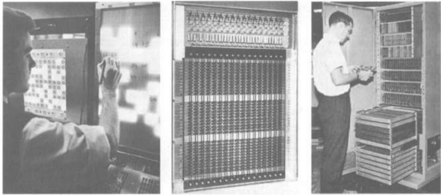
Resim 4.8. MINOS II: Operatörün görüntü kartı (solda), tek başına bir ağırlık çerçevesi (ortada) ve mantık devreleriyle birlikte ağırlık çerçeveleri (sağda). (Fotoğraflar, SRI International'ın izniyle kullanılmıştır.)
