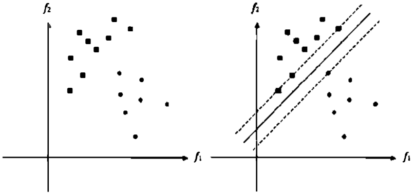
Resim 29.17. İki boyutlu uzamda noktalar ve doğrusal ayıran sınırlar.
