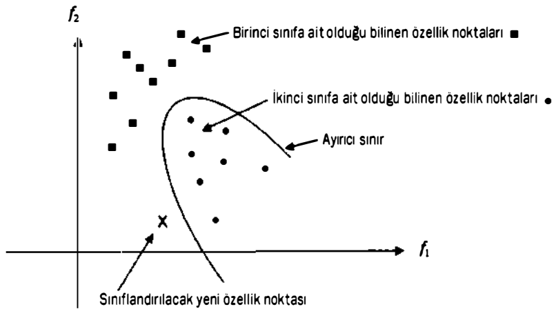
Resim 4.11. Özellik noktalarının ve ayırıcı sınırın iki boyutlu uzayı.
