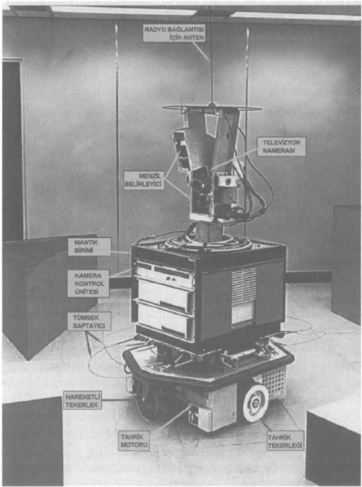
Resim 12.3. Shakey, Kasım 1968'deki haliyle (bazı bileşenleri etiketlenmiş). (Fotoğraf, SRI International'ın izniyle.)
