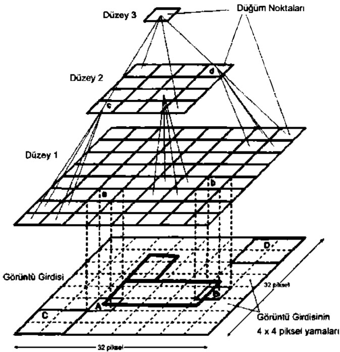
30.13. HZB modeli (Dileep George'un izniyle kullanılmıştır).
