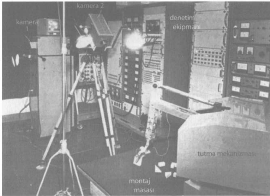
Resim 10.4. Hitachi'nin HIVIP robot montaj sistemi.
