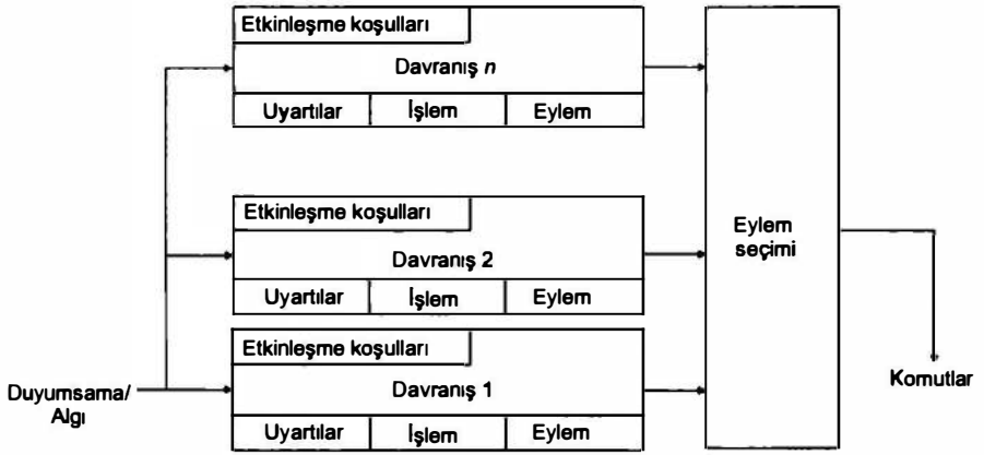
Resim 31.3. Davranış tabanlı mimari.
