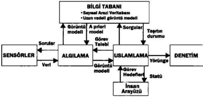
Resim 23.3. Martin Marietta'nın ALV'si (üstte) ve sistem yapılanması (altta). (ALV fotoğrafı DARPA'nın izniyle; diyagram: R. Terry Dunlay, "Obstacle Avoidance Perception Processing for the Autonomous Land Vehicle", Proceedings of the IEEE Robotics and Automation Conference, Los Alamitos, CA: CS Press, 1988, s. 912-917.)
