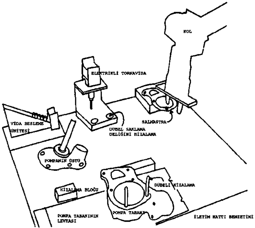
Resim 10.3. Su pompası montaj düzeneği. (Çizim, Robert Bolles'in izniyle kullanılmıştır.)
