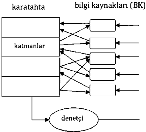
Resim 17.5. Karatahta mimarisi.
