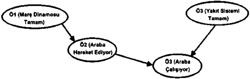
Resim 28.2. Ağ gösterimi.
