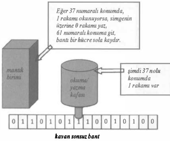
Resim 2.19. Turing makinesi
