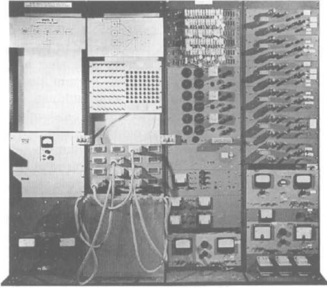
Resim 4.7. MINOS. Girdi anahtarlarına ve donanımın soldan ikinci rafında duran bunların işaret ışıklarına dikkat edin. Manyetik ağırlıklar, üçüncü rafın üst kısmındadır. (Fotoğraf, SRI International'ın izniyle kullanılmıştır.)
