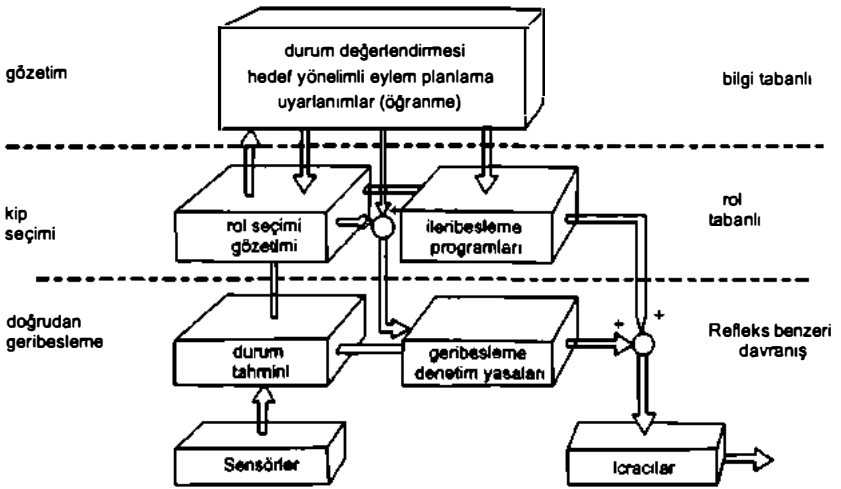
Resim 31.2. Sürücüsüz arabanın üç katmanlı mimarisi. (Ernst D. Dickmanns izniyle kullanılmıştır.)
