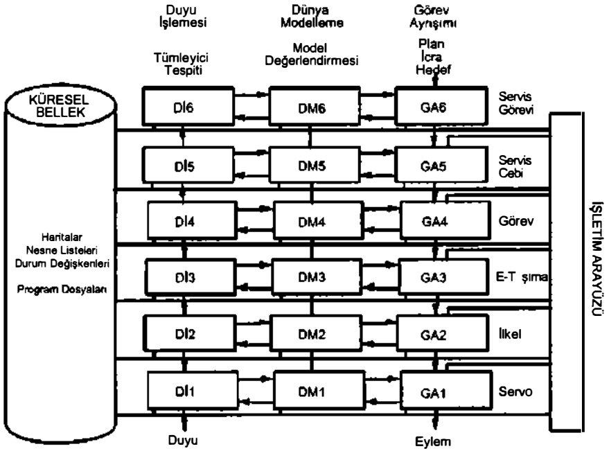
Resim 31.5. NASREM mimarisi. (Şu makalenin ikinci resminden: James S. Albus, "A Reference Model Architecture for Intelligent Systems Design", An Introduction to Intelligent and Autonomous Control , İkinci Bölüm, P. J. Antsaklis ve K. M. Passino (ed.), Dordrecht: Kluwer Academic Publishers, 1993, s. 27-56.)
