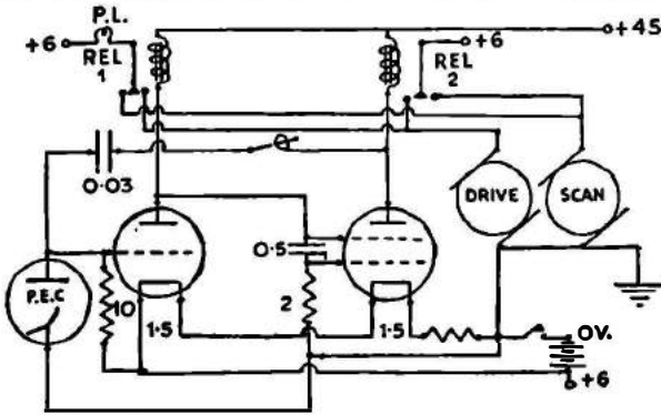
Resim 2.11. Grey Walter (üstte solda), Machina speculatrix 'i (üstte sağda), devre diyagramı (altta). (Grey Walter fotoğrafı şu kitaptan alınmıştır: Hans Moravec, ROBOT , Bölüm 2: Caution! Robot Vehicle!, s. 18, Oxford: Oxford University Press, 1998; "Tosbağa" fotoğrafı, Ulusal Amerikan Tarihi Müzesi, Smithsonian Enstitüsü'nün izniyle; devre diyagramı şu kitaptan alınmıştır: W. Grey Walter, The Living Brain , s. 200, Londra: Gerald Duckworth & Co., Ltd., 1953.)
