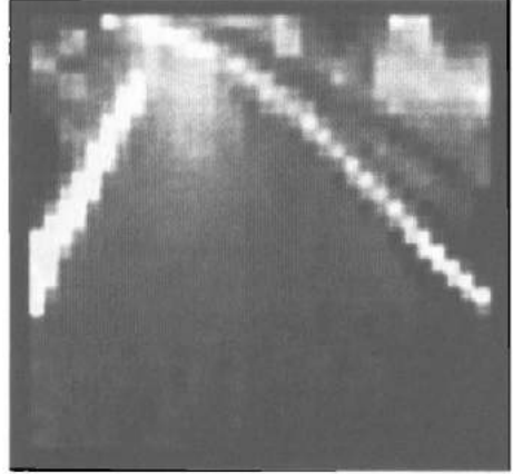
Resim 29.9. ALVINN ağı (solda) ve tipik yol imgesi (sağda) (Dean A. Pomerleau, "Neural Network Vision for Robot Driving", The Handbook of Brain Theory and Neural Networks içinde, Michael Arbib (ed.), Cambridge, MA: MIT Press, 1995. Bu makalenin bir versiyonu şu internet adresinde: http://www.ri.cmu.edu/pub_files/pub2/pomerleau_dean_1995_1/pomerleau_dean_1995_1.pdf .)
