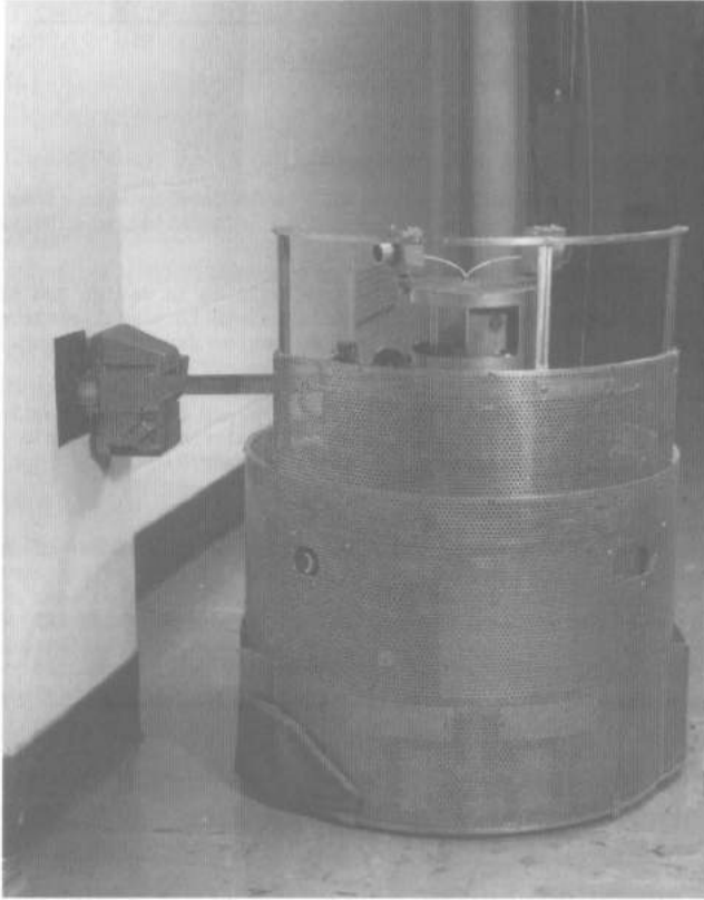
Resim 12.1. Johns Hopkins “Beast”i (Johns Hopkins Üniversitesi Uygulamalı Fizik Laboratuvarı’nın izniyle.)
