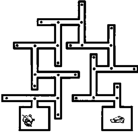
Resim 29.12. Labirent
