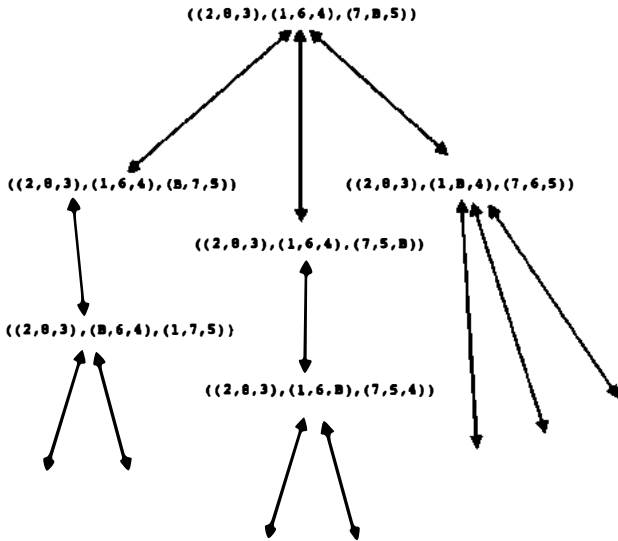
Resim 5.3. Arama ağacı.
