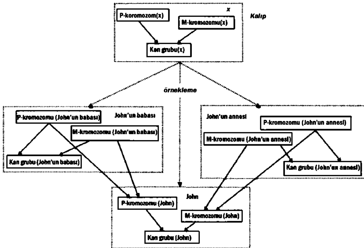
Resim 28.7. OİM örneği.
