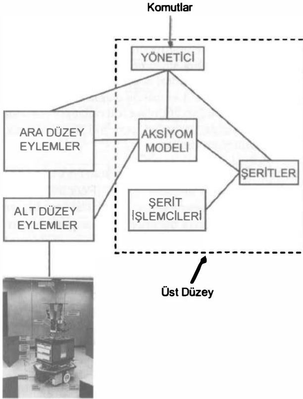
Resim 31.1. Shakey'nin üç düzeyli mimarisi.
