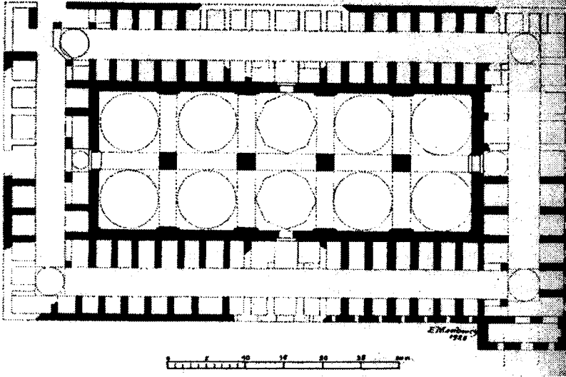
(Üstte) Mahmut Paşa Bedesteni'nden görünüş. (Altta) Bedestenin plâni. (Yanda) Anadolu Medeniyetleri Müzesi.
