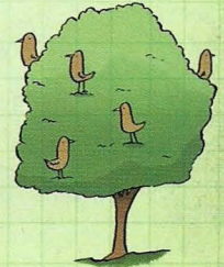
B ağacı
