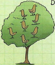
A ağacı
