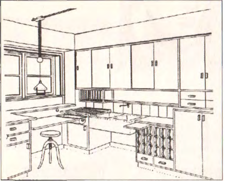
Resim 13 Schütte-Lihotzky'nin Frankfurt Mutfağı: Eşölçülü.
