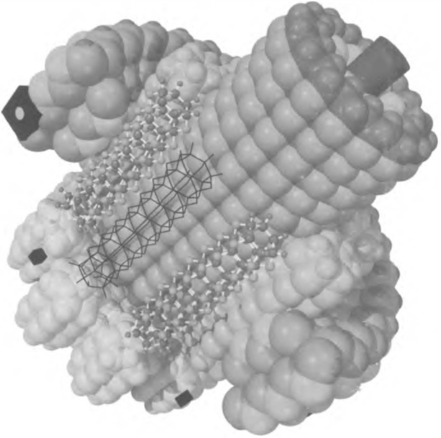
Şekil 10 Gezer dışı. Drexler tarafından tasarlanmış olan bu erken dönem gezer dışı çeşitlemesi, moleküler dinamik tekniği kullanılarak benzetimi yapılmış ilk nanomakine sistemidir.
