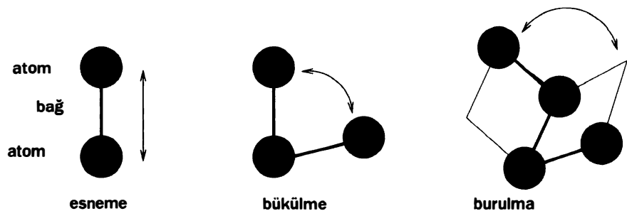
Şekil 6 Moleküler mekanik. Kovalent bağların üzerindeki ve arasındaki güçler. Bunlar, tıpkı moleküler mekanik güç alanlarıyla açıklanır.
