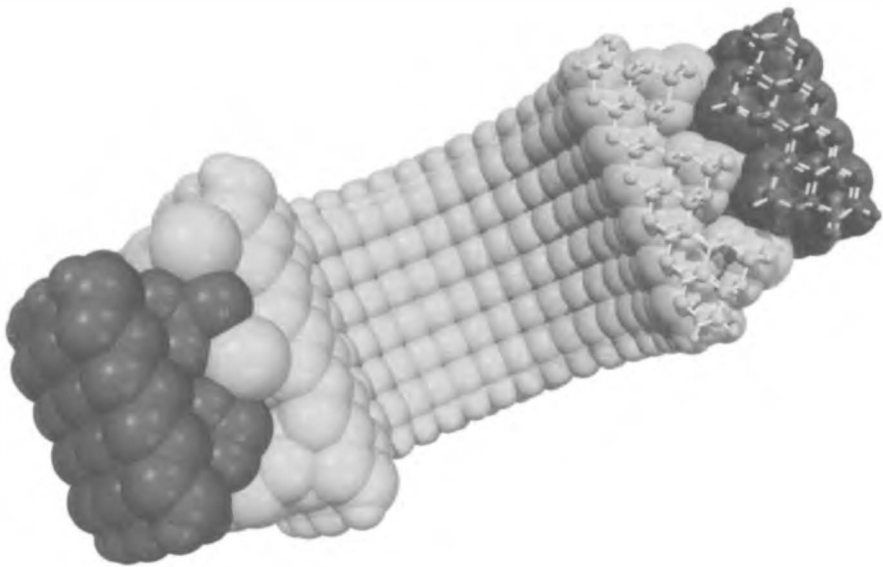
Şekil 9 Moleküler bir silindirik rulman. Drexler'ın bu büyük-elmas tasarımı hem dikey hem de yatay eksenlerde hatırı sayılır bir bükülme direnci sergiler. Büyük topraklar, atomların van der Waals yüzeylerini temsil ediyor; küçük topraklar ve çubuklar bağ yapılarını temsil ediyor.
