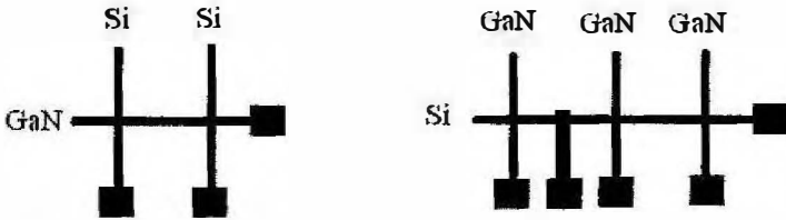
Silisyum (Si) ve galyum nitrür (GaN) nanotellerden yapılmış “ve”, “veya” mantık devre örnekleri (şematik).
