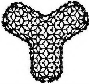
Karbon nanotüp eklemlerinde altıgenden başka beşgen ve yedigen geometri de görülür.
