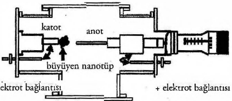
Karbon nanotüp üretme yöntemlerinden ark yöntemi.
