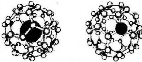
Katkılandırılmış karbon top modelleri. Soldaki şekilde başka bir atom karbon-60'ın içine yerleştirilmiş, sağdaki şekilde ise karbon atomlarından birinin yerine başka bir atom yerleştirilmiş.
