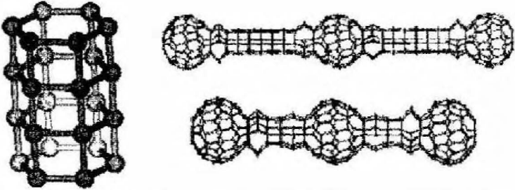
Benzoçubuk modeli ile benzoçubuklarla bağlanmış karbon-60 topları.
