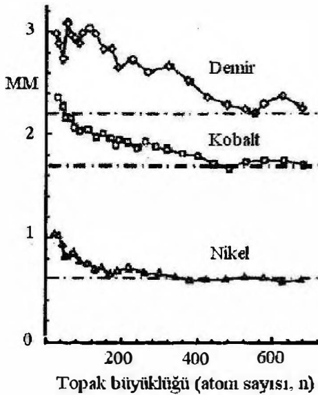
Demir, Kobalt ve Nikel topaklarında atom başına düşen manyetik momentin (MM) topak büyüklüğüne göre değişimi. Yatay kesikli çizgiler kristal değerini gösteriyor.
