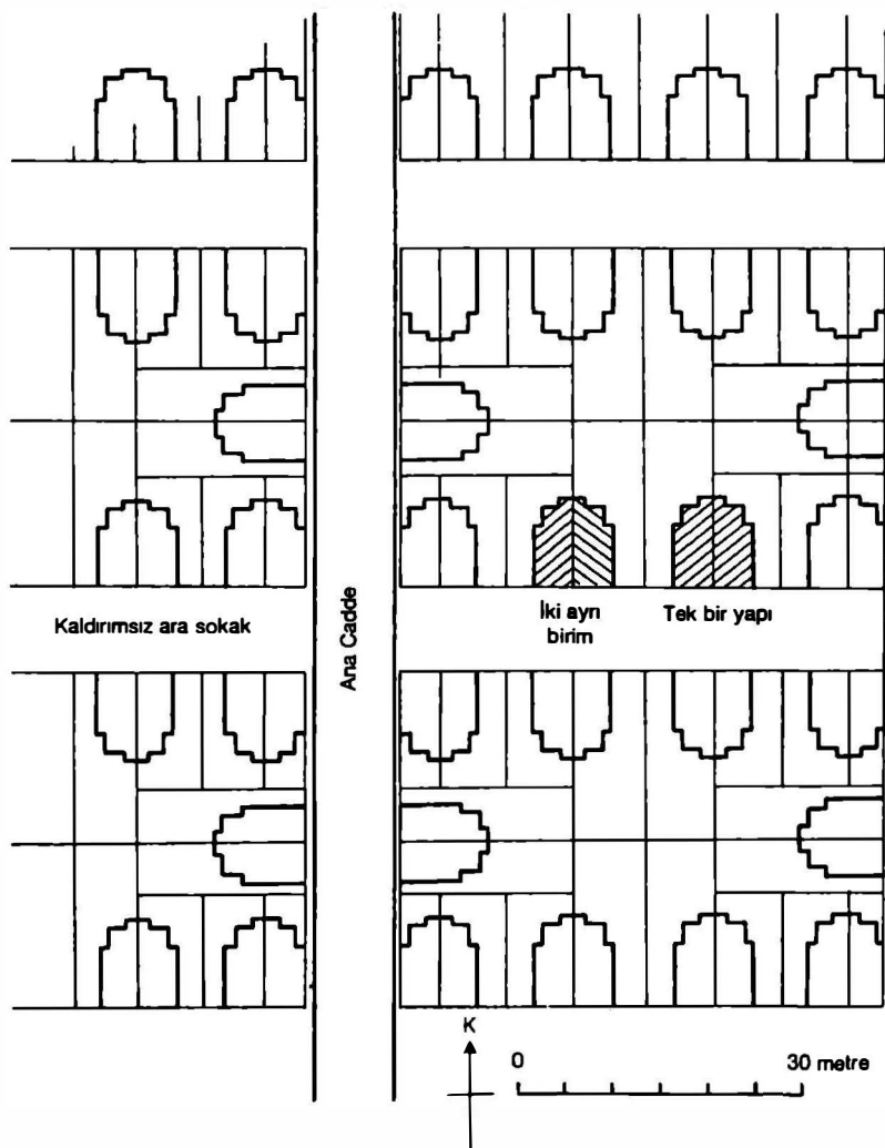
Şekil 1. Yanya: Sokak ve evlerin planı.
