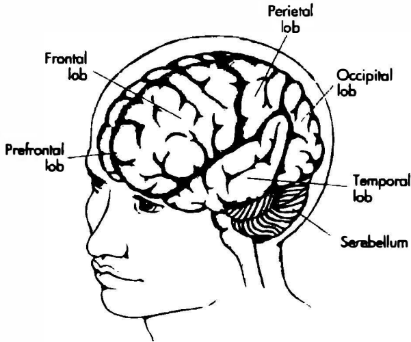
Şekil E Beyincik (serebellum) ve beyin yarıküresinin (serebral hemisfer) başlıca bölümlerini gösteren beyin sol yanının görüntüsü.
