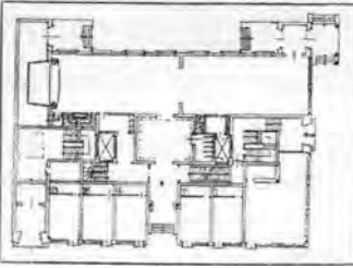
Birinci mükâfat. Kat planları.
