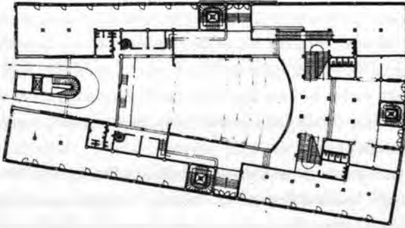
Röhlöve 9. Ankara, İkinci Vakıf Hanı, yer katı planı
