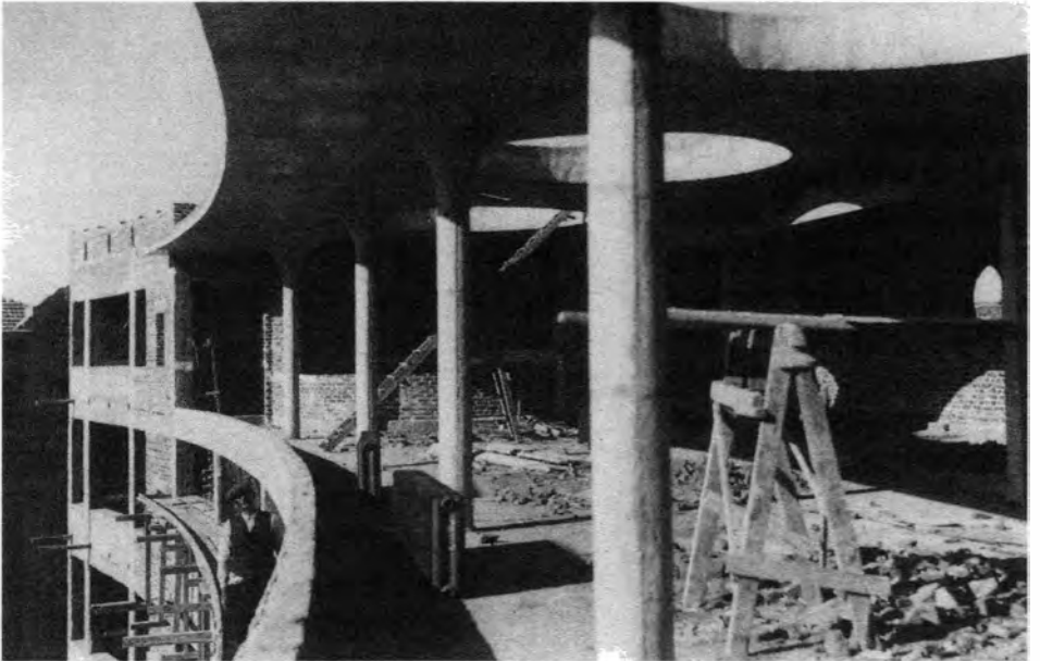
3.18 Martin Elsaeser'in yaptığı Sümerbank binasının inşaat fotoğrafları. Üst: Mayıs 1937, inşaat yarılanmış durumda, kale etrafındaki Eski Ankara'nın kentsel dokusu karşısında binanın ne kadar dev ölçekte kaldığı görülüyor. Alt: İnşaat halindeki üst katın Eylül 1937'deki görünüşü, betonarme mantar sütunlar ve çatıda dairesel ışık delikleri dikkat çekiyor (Sümerbank mimarlık bürosu arşivleri, Ankara).
