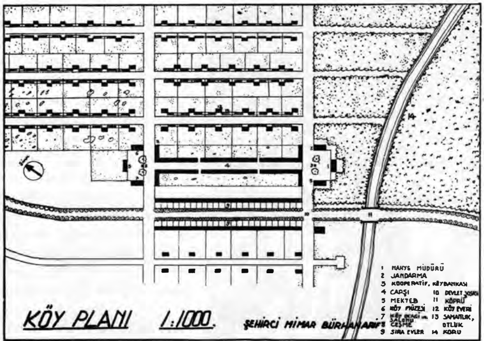
2.27 "Şehirci mimar" Burhan Arife ait, tekbiçimli ızgara planlı örnek köy projesi (1935) (Arkitekt 5, no. 11-12, 1935).
