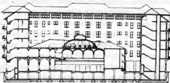
Röhlöve 10. Ankara, İkinci Vakıf Hanı, boyuna kesit
