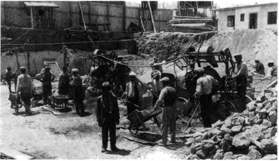
4.13 Sümerbank binasının inşaatı, Ankara (1937). Fotoğraf, bu büyüklük ve önemdeki bir bina için bile inşaat sanayinin ne kadar ilkel koşullarda olduğunu gösteriyor (Sümerbank mimarlık bürosu arşivleri, Ankara).
