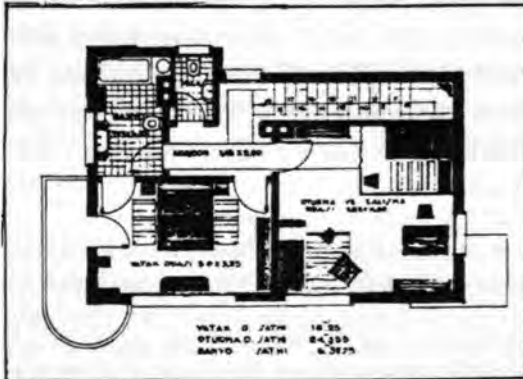
4.1 Bir öğrencinin müstakil ev projesi (1930); Ernst Egli'nin Sanayi-i Nefise'deki stüdyosunda mimarlık öğrencisi olan Edip Hikmet'in çalışması. Düz çatılar, konsollar, yuvarlak balkonlar, yatay şerit pencereler ve tezyinat yokluğu, halk arasında "kübik mimari" olarak tanınan "Yeni Mimari"nin karakteristik özellikleriydi ( Mimar 1, no. 1, 1931).
