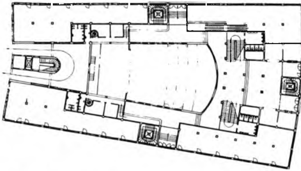
Rölöve 9. Ankara, İkinci Vakıf Hanı, yer katı planı
