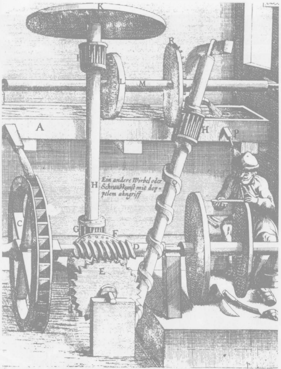
Şekil 48. Bıçak bilemekte kullanılan sürekli hareket makinesi. Georg Andreas Böckler, Theatrum Machinarum Novum , Nüremburg, 1673.
