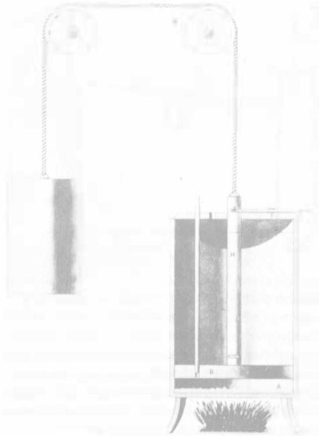
Şekil 99. Papin'in buhar makinesi.
