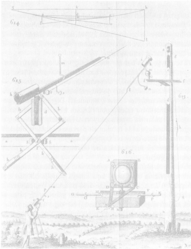
Şekil 75. Huygens'in havai teleskopu
