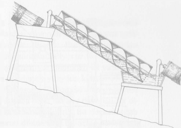
Şekil 21. Archimedes burgusu. Birbirine eklenmiş bir dizi Archimedes burgusundan oluşan bir düzenele oldukça dik yamaçlardan yukarı su taşılabiliyordu.
