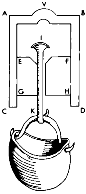
Şekil 87. Galileo'nun vakumun oluşmasına karşı direnci ölçme deneyi için yaptığı alet. İçi boş silindir (AD) içinde yer alan tahta pistonun (EH) üzerindeki boşluğa su konmakta, çengele asılı kova ise ağırlaşıp aşağı inmeye başlarken kumla doldurulmaktadır.
