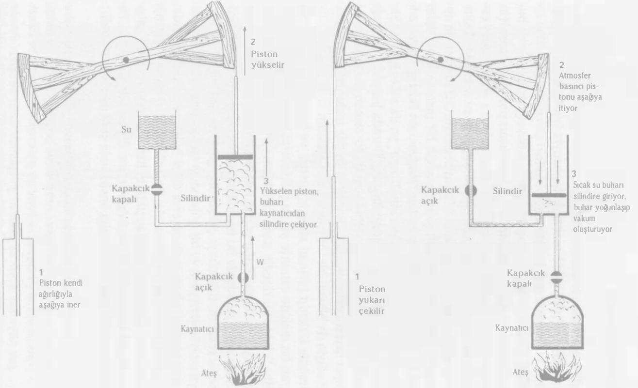
Şekil 101. Newcomen'in buhar makinesi.
