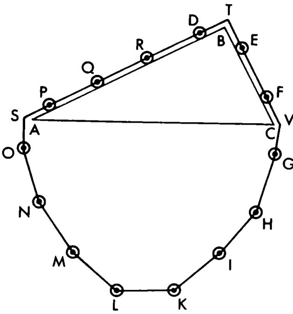
Şekil 64. Dikaçılı prizma üzerinden sarkıtılmış sürtünmesiz zincir halka,
