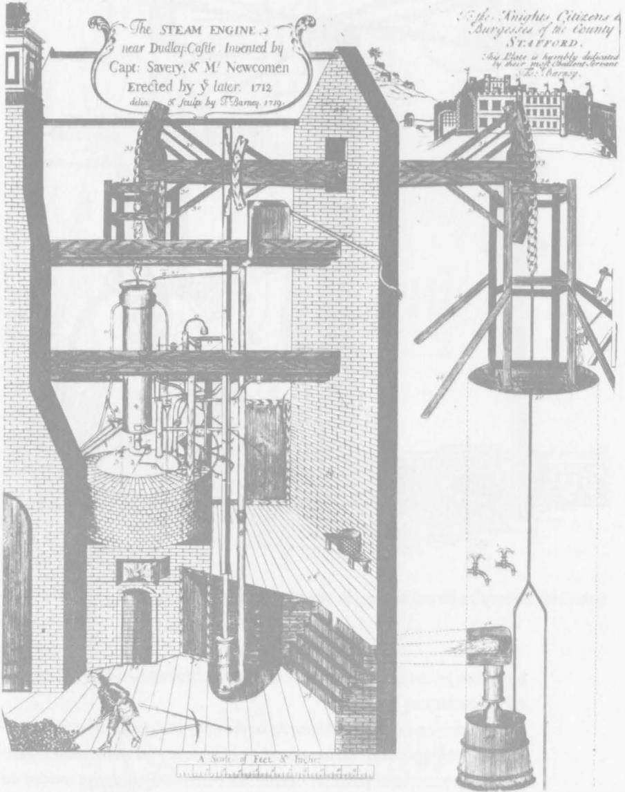
Şekil 103. 1712'de Dudley Castle yakınlarında kurulan Newcomen buhar makinesi- ni gösteren bu resim 1719'da Barney tarafından oyma klişe yöntemiyle yapılmıştır.
