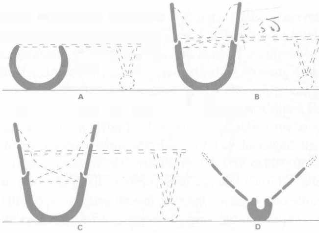
Şekil 7. İçi oyulmuş kütükten yapılan kayıklarda omurganın geliştirilmesini gösteren kesitler. (A) İçi oyulmuş kütük; (B) Bir kat yan tahta eklendikten sonraki görünüm; (C) İkinci kat yan tahtaların eklenmesi; (D) Omurganın geliştirilmiş durumu.
