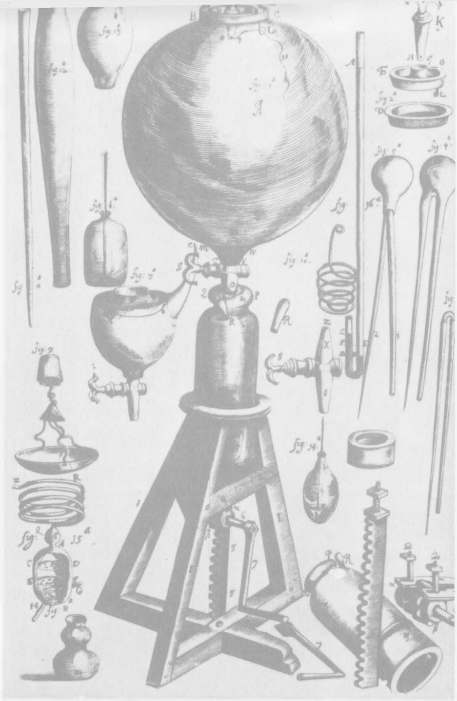
Şekil 94. Boyle'un hava pompası ve cam küreden oluşan düzeneği.
