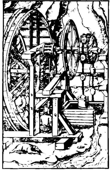
Şekil 53. Ayakla döndürülen çark ve zincirli tulumbadan oluşan diğer bir düzenek. G. Agricola, De re metallica , Basel, 1556.
