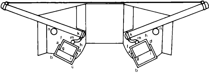
Şekil 24. Basıncı hava ile çalışan bir mancınık. Çizimin Ctesibus'a ait olduğu sanılmaktadır. M.Ö. Birinci Yüzyıl.
