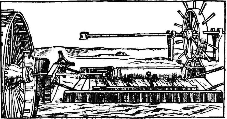
Şekil 60. Top namlusunun içinin oyulması. Biringuccio, De la Pirotecnia , Venedik, 1540
