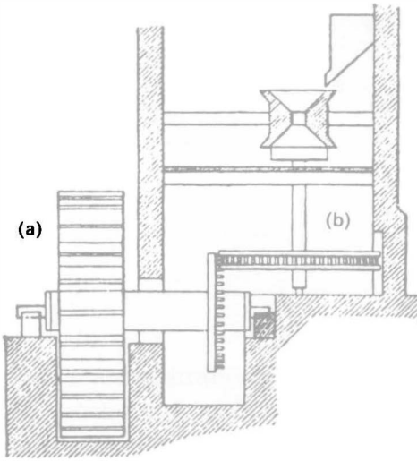
Şekil 22. Roma döneminden kalma su değirmeni. Vitruvius'un bir çiziminden alınmıştır.
