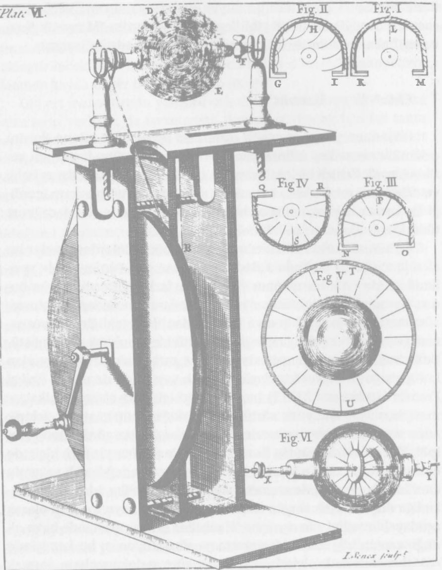
Şekil 106. Hauksbee'nin iplik bükme makinesini kullanarak cam kürenin içindeki havayı boşaltma deneyi (1714).
