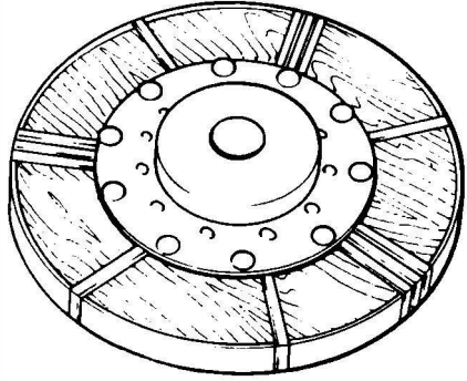
Şekil 11. Çivili tekerlek. Susa (Mezopotamya), M.Ö. 2500.
