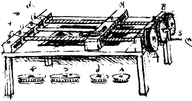
Şekil 47. Burgu tornası. Da Vinci .
