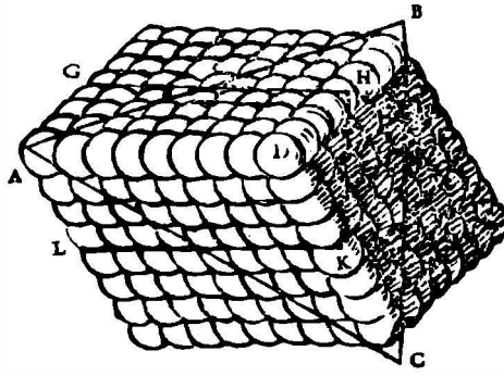
Şekil 84. Huygens'in İzlanda spatını oluşturan rombik formları gösteren çizimi.
