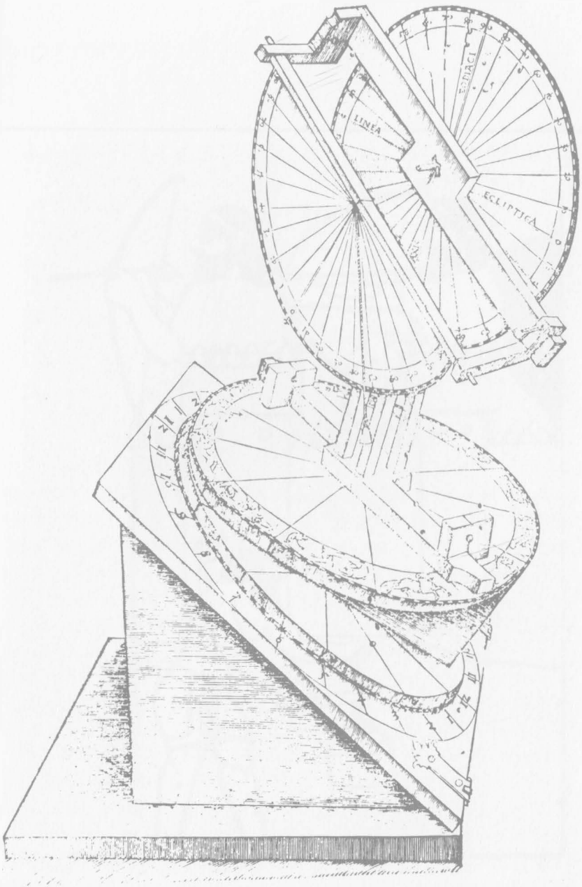
41. Astronomik gözlemde kullanılan üzeri derecelendirilmiş çemberler.
