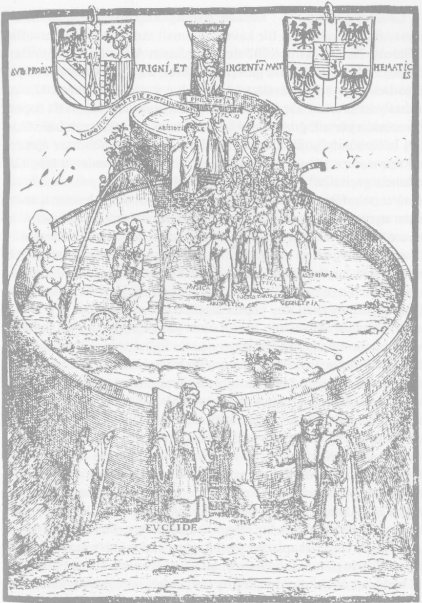
Şekil 63. Yeni Bilim kavramı, Nicolo Tartaglia, Nova Scientia , Venedik, 1537.
