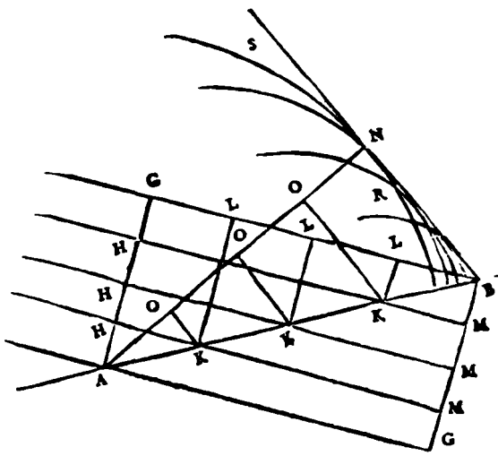
Şekil 82. Huygens'in ışığın yansımısını gösteren çizimi.
