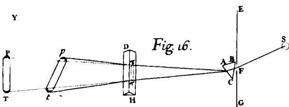
Şekil 78. Newton'un Opticks 'inden alınan, ışığın kırılığını gösteren deneyler.
