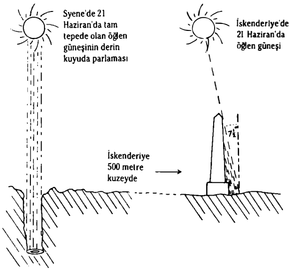
Şekil 27. Eratosthenes'in Dünya'nın çevresini ölçme yöntemi. Syene'de Yaz Dönümünde güneşin tam tepe noktasında bulunmasına karşılık İskenderiye'de güneş ışınlarının "dikey" e göre 7 \frac{1}{2} (derece işareti konulacak) eğiklik gösterdiğini farkedenden ve bu iki nokta arasındaki uzaklığı ölçen Eratosthenes buradan yola çıkarak Dünya'nın çevresini 250.000 stadia (yaklaşık olarak 36.000 km.) olarak hesaplamıştır.
