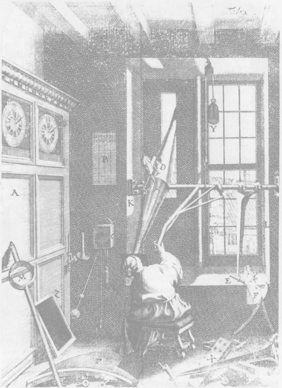
Şekil 69. Römer teleskopu. Peder Horrobow'un Basis Astronomiae Harniae 'sinden (1735).
