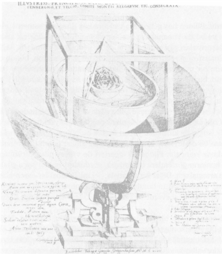
Şekil 58. Kepler'in gezegenlerin hareketlerine ilişkin ilk yorumu. De Harmonice Mundi , Linz, 1619.
