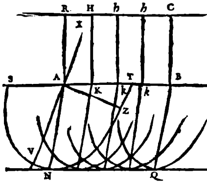
Şekil 83. Huygens'in ışığın İzlanda spatı içindeki davranışını gösteren çizimi.
