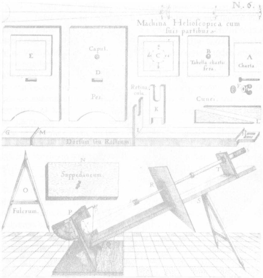
Şekil 73. Scheiner'in helyoskopu, 1630.
