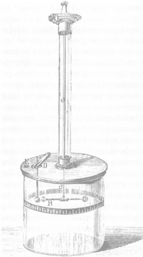
Şekil 108. Coulomb'un tor- siyometresi.
