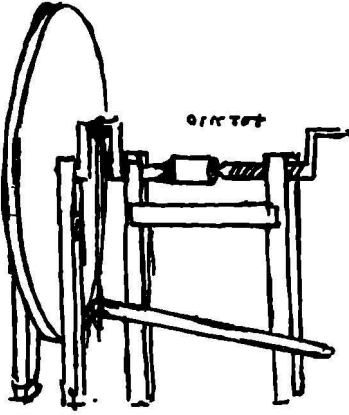
Şekil 44. Volanlı torna. Leonard da Vinci'nin Codice Atlantico 'sundan.
