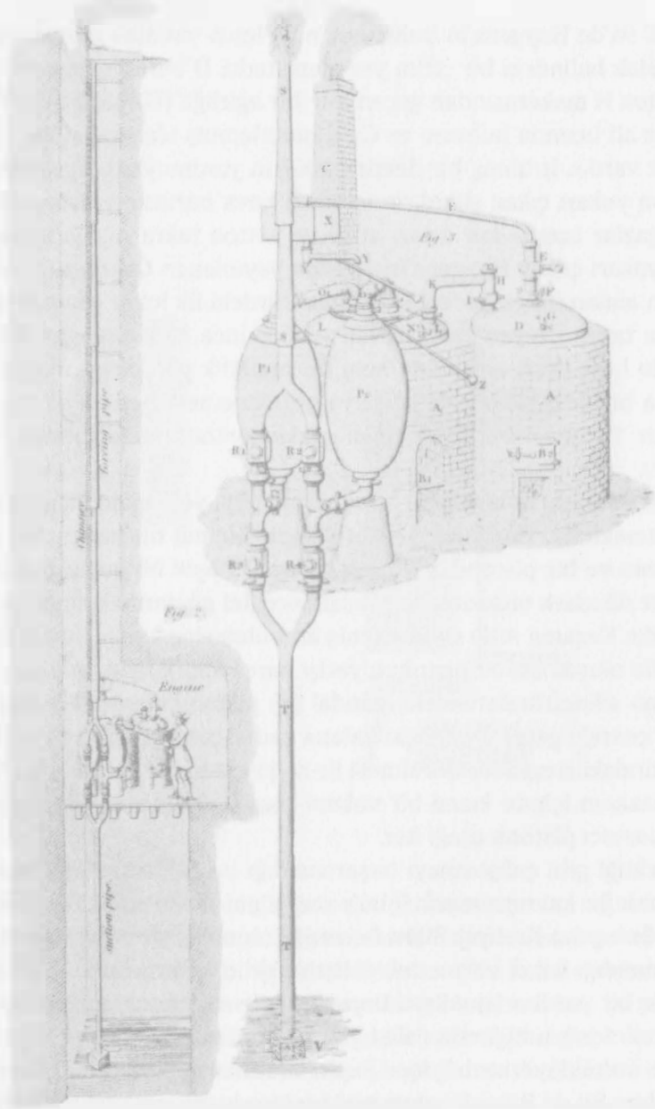
Şekil 100. Savery'in "Madencinin Dostu ya da Suyu Ateşle Boşaltan Makine" si. Farey, Treatise on the Steam Engine .
