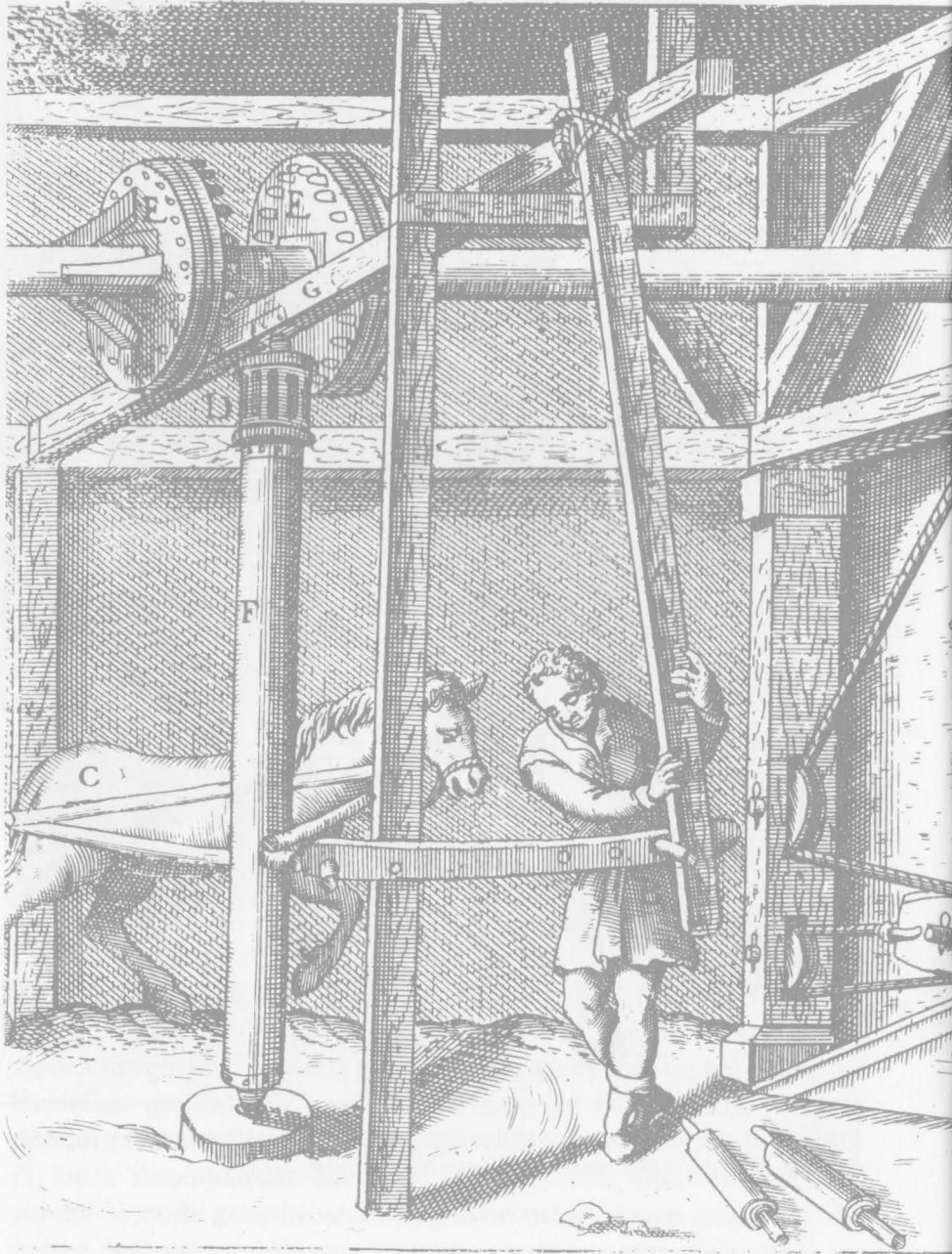
Şekil 49. Yarı-mekanik haddehane. Zonca, Nuova Teatro di Machine et Edificii , Padua, 1607.
