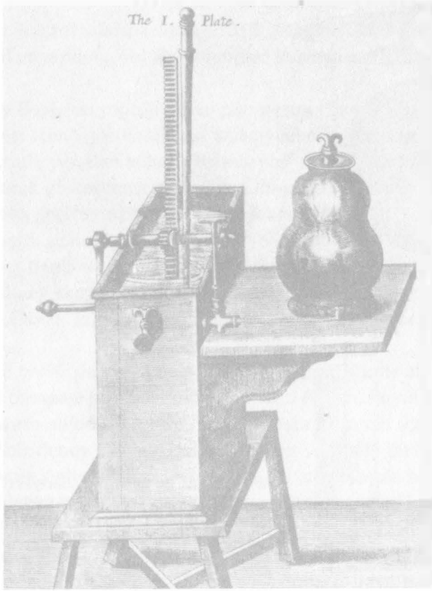
Şekil 95. Boyle'un ikinci hava pompası.
