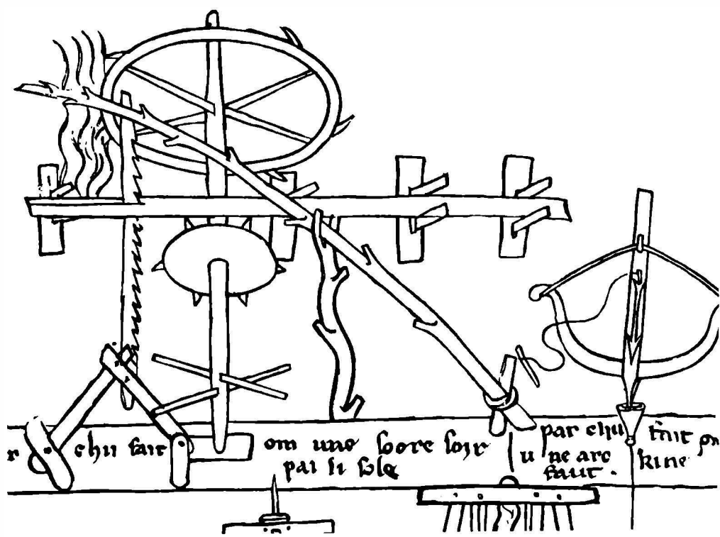
Şekil 31. Su gücü ile çalışan bıçkı makinesi. Villard de Honnecourt, 1250.
