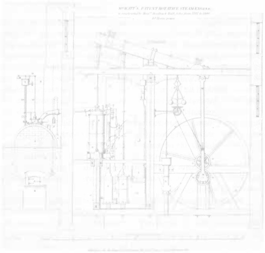
Şekil 105. Watt'ın çift yönlü çalışan rotatif buhar makinesi. Resmin sağında Güneş-gezegen dişlisi görülmektedir.
