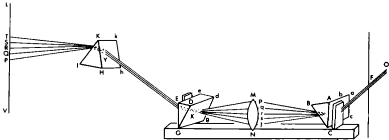
Şekil 77. Newton'un spektral renklerin tekrar birleşip beyaz ışık oluşturduğunu gösteren deneyi.
