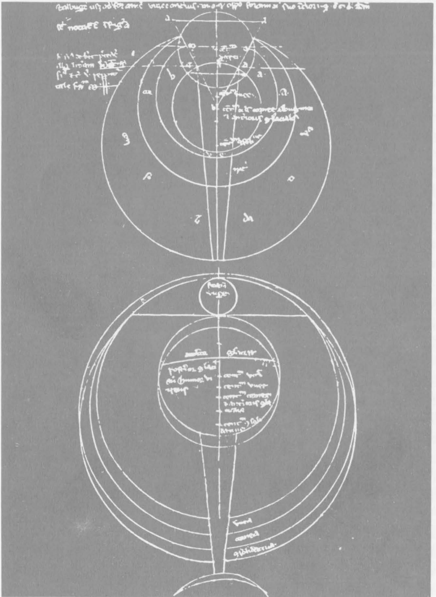
Şekil 28. Gözün kırılım işlevini anlatan bu şema Roger Bacon'un Opus Majus 'undan alınmıştır (M.S. 13 üncü yüzyıl)
