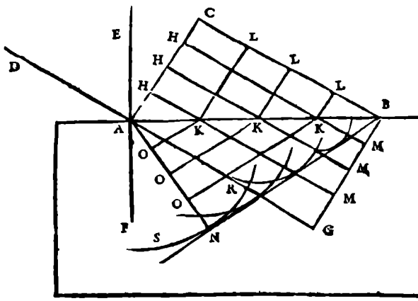
Şekil 81. Huygens'in ışığın kırılımı gösteren çizimi.
