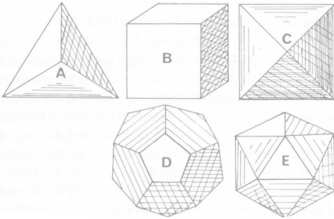
Şekil 25. Beş geometrik cisim: (A) Tetrahedron (dört yüz); (B) Küp (altı yüz); (C) Oktahedron (sekiz yüz); (D) Dodekahedron (on iki yüz); (E) İkosahedron (yirmi yüz). Her cisimde tüm yüzler yüzey ve biçim yönünden birbirine eşittir.
