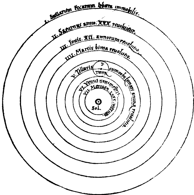
Şekil 55. Copernicus'un Evreni. De Revolutionibus orbium coelestium (1543). (I) Sabit yıldızların küresi; (II) Satürn'ün yörüngesi; (III) Jüpiter'in yörüngesi; (IV) Mars'ın yörüngesi; (V) Dünya ve Ay'ın yörüngesi; (VI) Venüs'ün yörüngesi; (VII) Merkür'ün yörüngesi. Merkezde güneş yer almaktadır.
