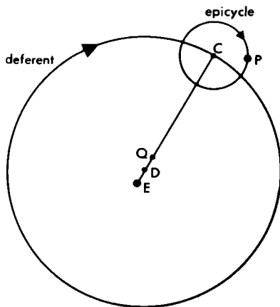
Şekil 54. Episiklik yörünge. P gezegeni, D deferentin merkezini, E Dünya'yı göstermektedir. Episikliğin merkezi C , D 'nin çevresinde düzgün bir yol izlemeyip CQ çizgisinin eşit zamanlarda eşit açılardan geçmesini sağlayacak biçimde hareket eder.
