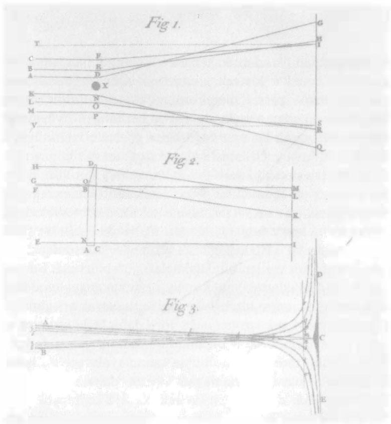
Şekil 86. Newton'un Opticks 'inden ışığın kırınımını gösteren çizim.
