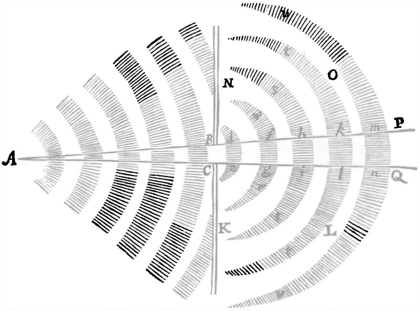
Şekil 79. Newton'un Principia 'sından ışık parçacıklarını gösteren şema.
