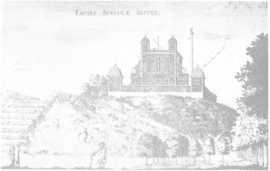
Şekil 70. Greenwich Kraliyet Gözlemevi
