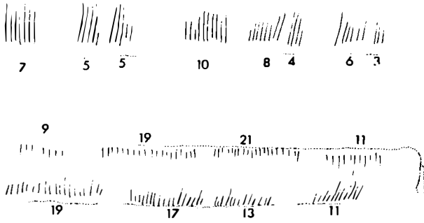
Şekil 2. Yaklaşık 12.000 yıl önce asal sayıların ve çarpım işleminin bilindiğini gösteren, üzerinde çentikler açılmış kemik parçası (Ishango, Güney Afrika).
