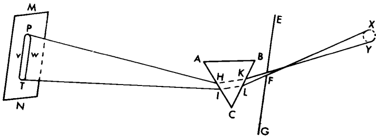
Şekil 76. Kraliyet Bilim Derneği'nin periyodik yayınlarından alınmış olan bu çizim Newton'un ışık spektrumunu göstermektedir.
