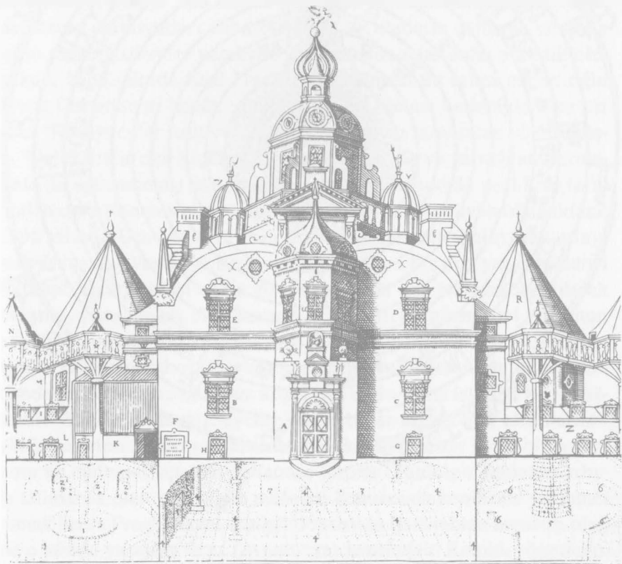
56. Tycho Brahe'nin Uranienborg Gözlemevi.
