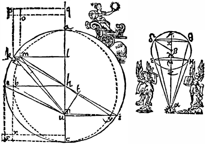
Şekil 59. Kepler'in Mars'ın eliptik yörüngesini gösteren çizimi. Astronomica Nova , Prag, 1609.
