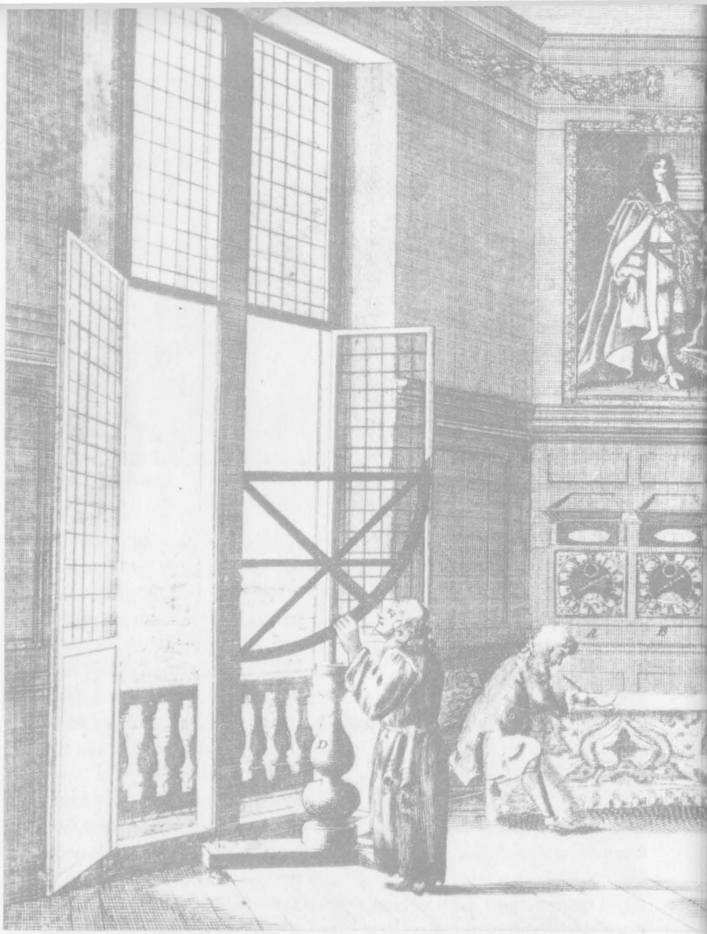
Şekil 71. Greenwich Gözlemevinde teleskop ve kuadrant ile gözlem yapan astronomlar.
