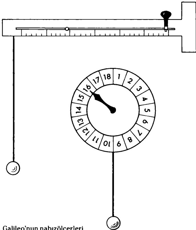
Şekil 65. Galileo'nun nabızölçerleri.
