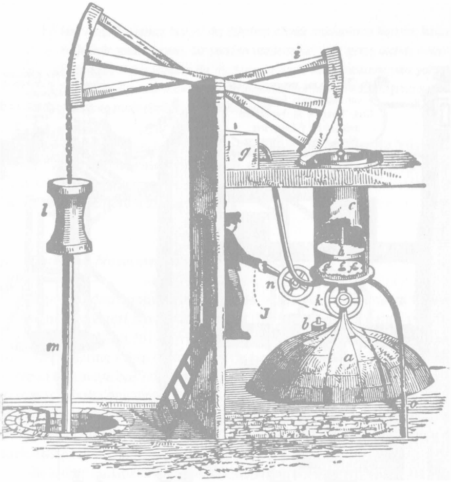
Şekil 102. Savery'in biracı kazanıyla yaptığı buhar makinesi.
