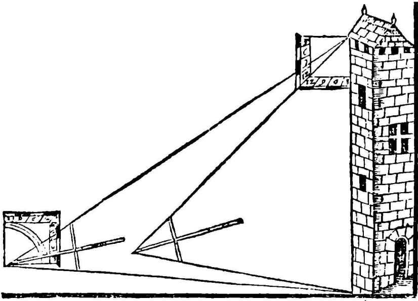
Şekil 39. Bir kulenin yüksekliğinin uzaktan ölçülmesi.
