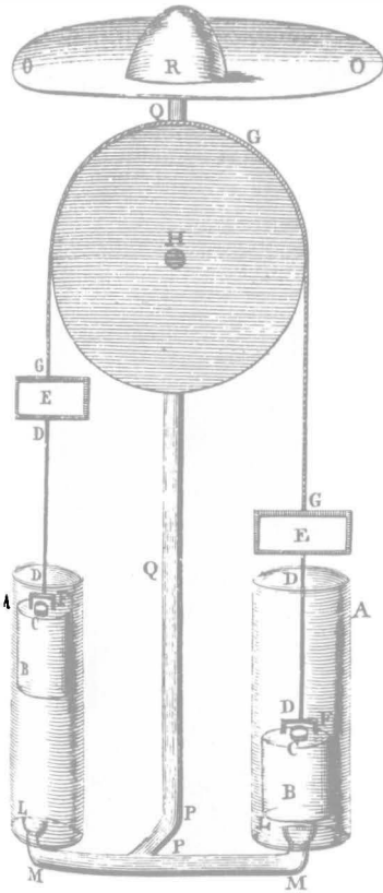
Şekil 96. Boyle'un ayak pedallarıyla (EE) çalıştırılan üçüncü hava pompası. O tablası üzerindeki R yarıküresinin içindeki havanın boşaltılması ile vakum oluşturulmaktaydı. The Works of R. Boyle , 1772
