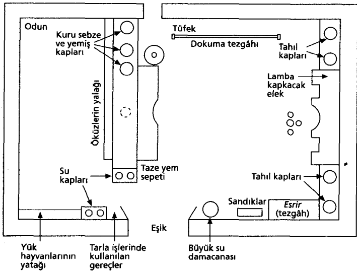
Kabiliye evinin planı. P. Bourdieu, Algeria 1960 'tan (Cambridge University Press/Maison des Sciences de l'Homme) alınmıştır.
