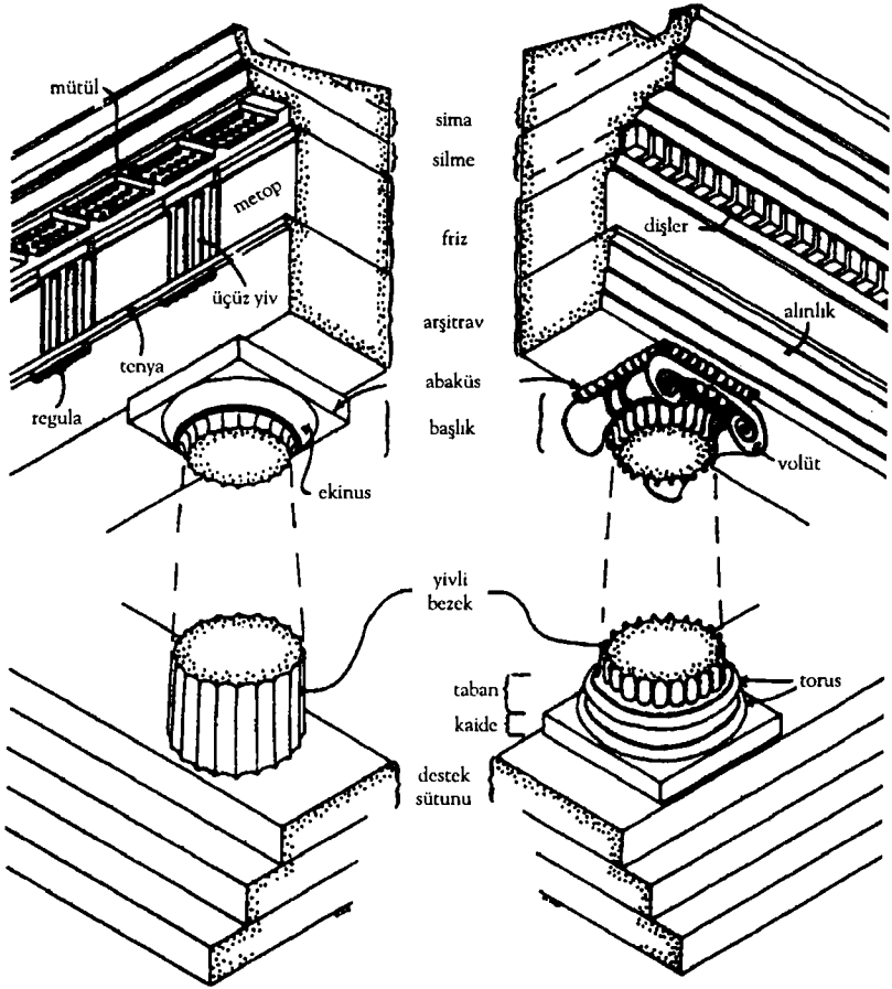
Dor ve İon düzenleri. Bu figür, bu iki özgün klasik düzen arasındaki temel farkları resmeder.
