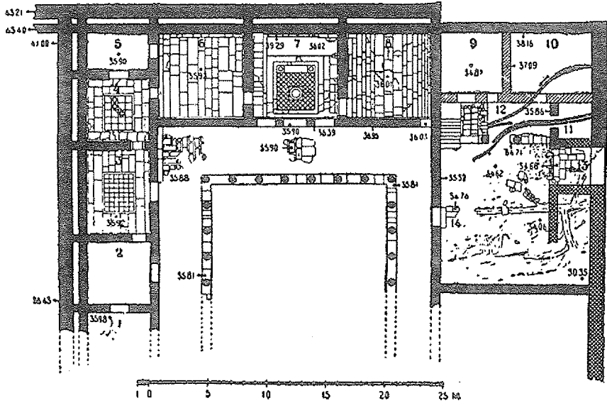
Mit. d. Deutsch Arch. Inst.'den 1903'te Bergama'da bulunan Yunan Evi'nin planı 13. Prothyron 7. Tablinum
