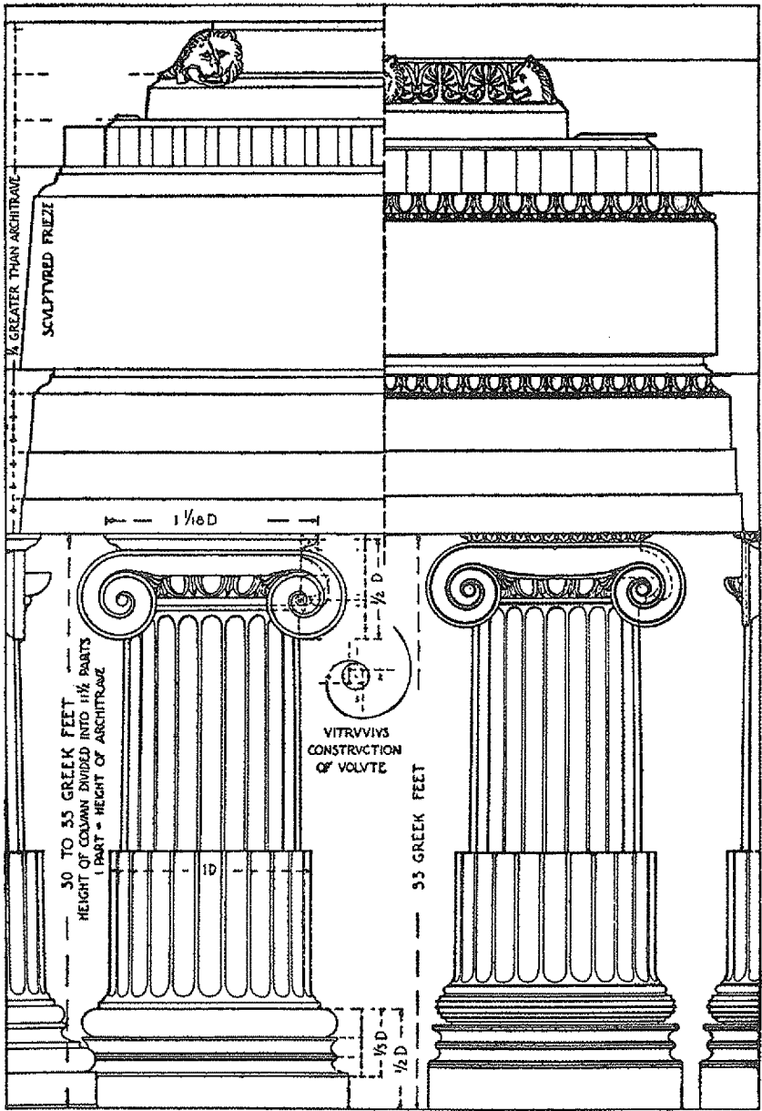
Vitruvius'a göre İyon düzeninin Halikarnas Mozalesinin sütun düzeniyle karşılaştırılması
