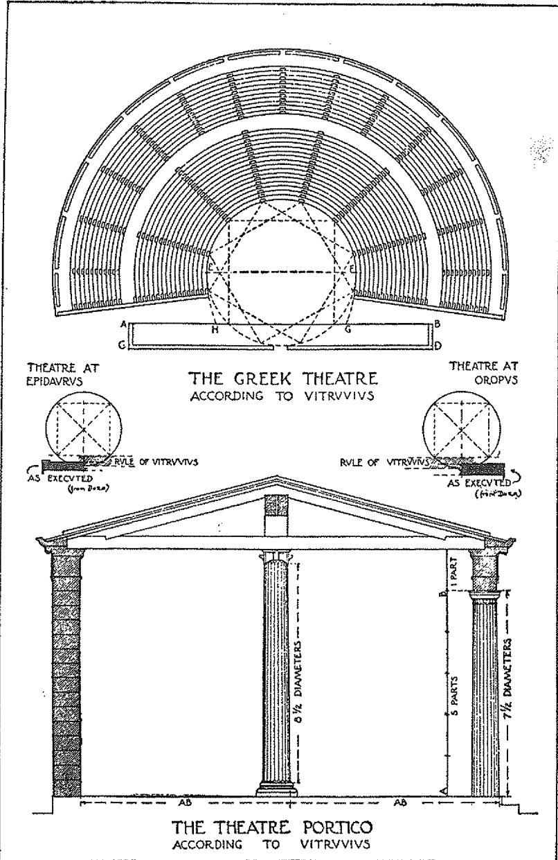
Vitruvius'a göre Yunan tiyatrosu
