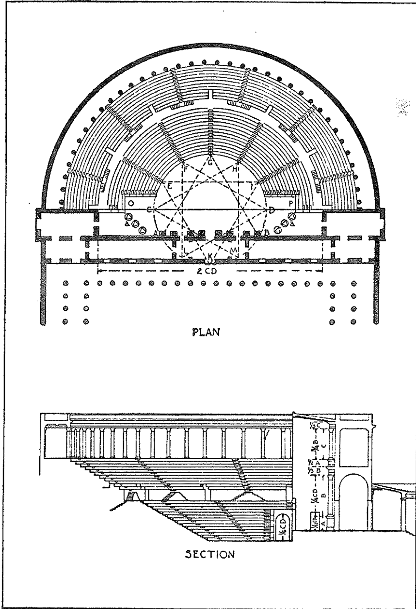
Vitruvius'a göre Roma Tiyatrosu
