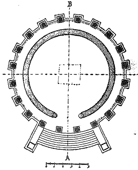
Durm'dan Roma'da Vesta Tapınağı'nın planı
