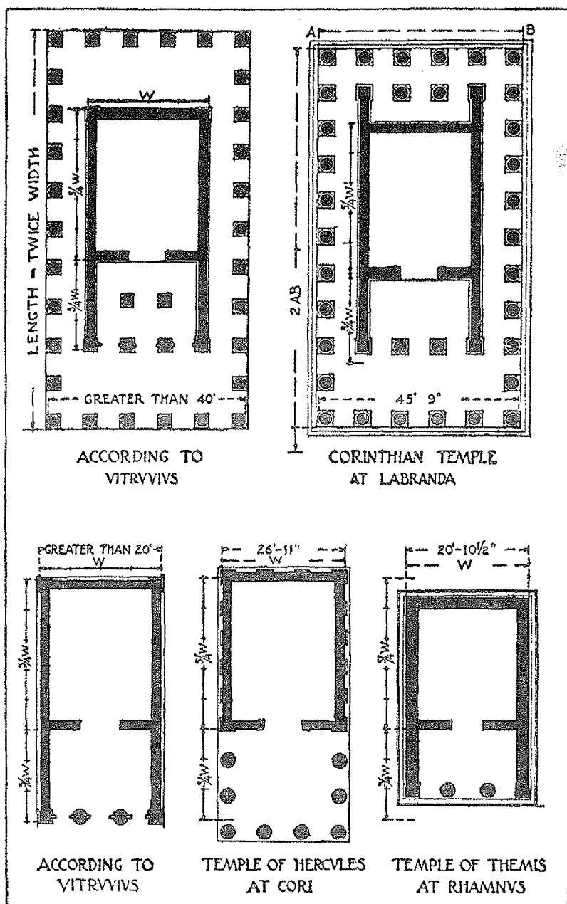
Vitruvius'un tapınak planının gerçek örneklerle karşılaştırılması
