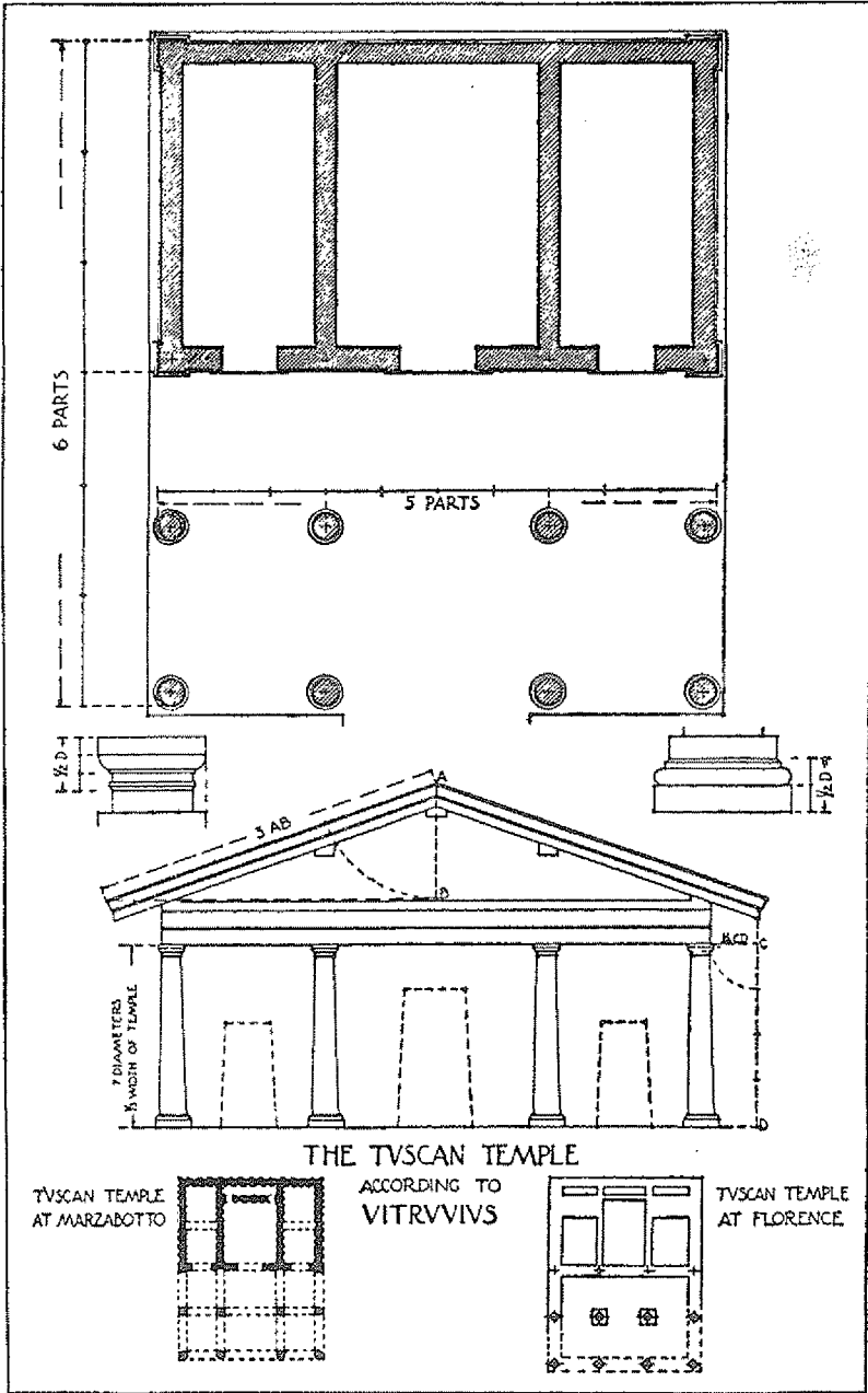
Vitruvius'a göre Toskana Tapınağı
