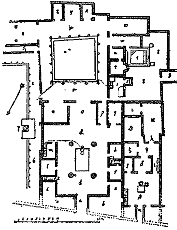
Mau'dan Gümüş Evliik Evi'nin planı, Pompeii
