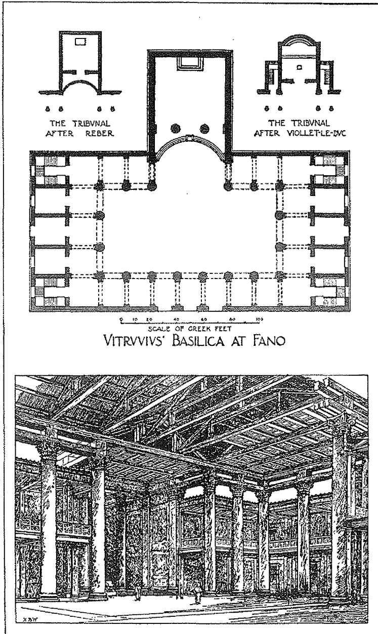
Vitruvius'un Fano'daki Bazilikası
