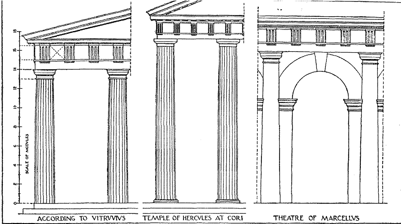
Vitruvius'un dor düzeninin Cori Tapınağı ve Marcellus Tiyatrosu ile karşılaştırılması
