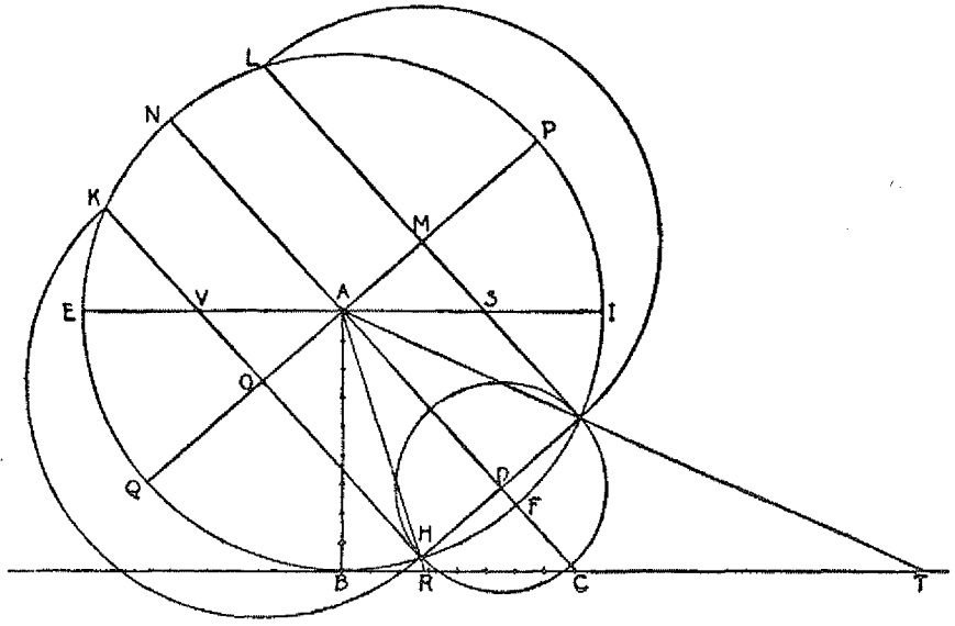
Analemmannın inşa edilmesi
