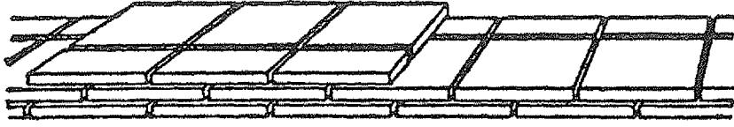
Reber'e göre Vitruvius'un tuğla örgüsü
