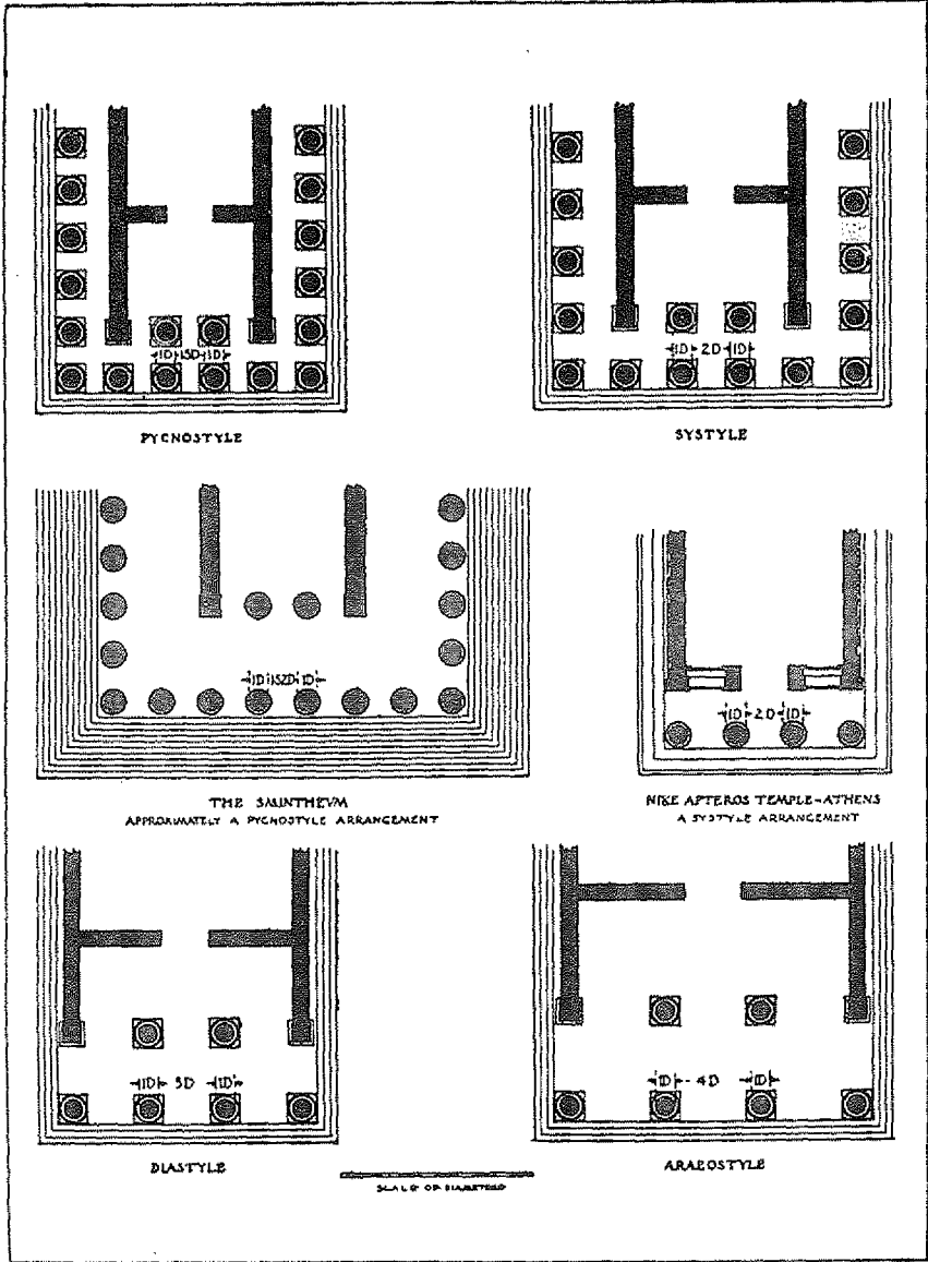
Tapınakların sütun aralıklarına göre sınıflandırılması
