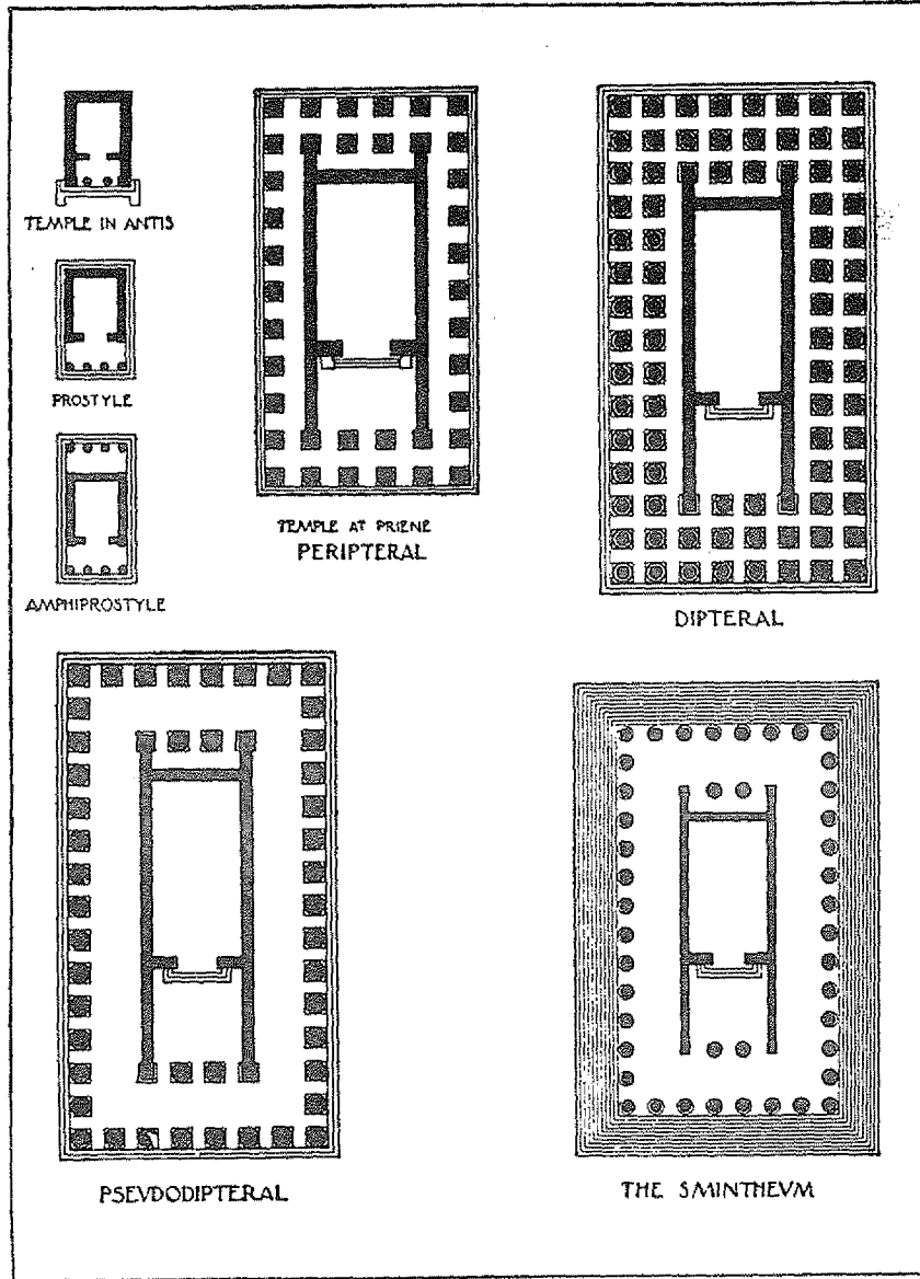
Sütün dizilerinin düzenlenmelerine göre tapınakların sınıflandırılması
