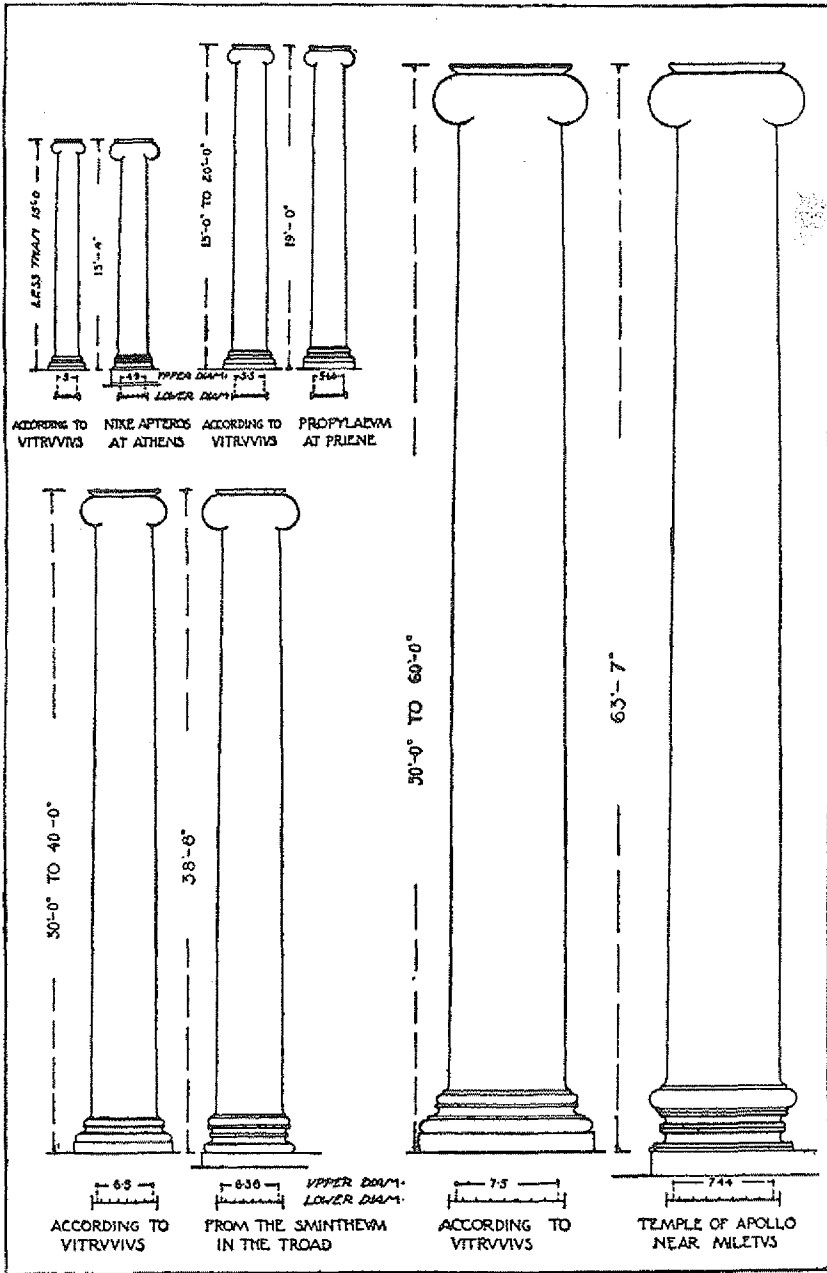
Sütunların yükseklik ölçülerine göre incelenmesi
