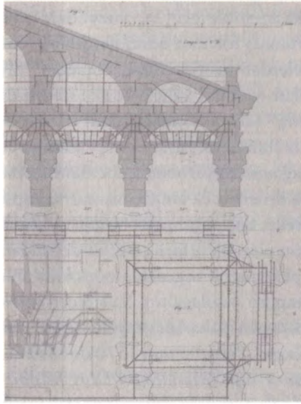
Görsel 10 Rondelet'in inşaat teknolojisine ilişkin kitabı teknik bilginin taşınabilir hâle gelişinde öncü yayınlardan biridir. Örnek: Paris'te Ste. Genevieve Kilisesi portikosunun demir donatı detayları.
