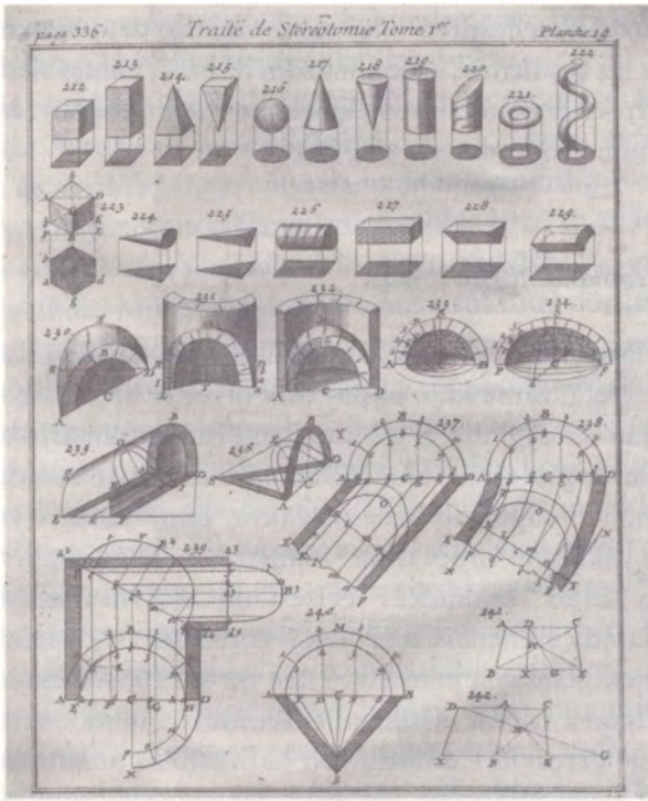
Görsel 12 Stereotomi (taş kesme bilgisi) mimarlığın matematiksellesmesinde önemli duraklardan biridir. Örnek: Amédée Frézier, La théorie et la pratique de la coupe des pierres et des bois pour la construction des voûtes et autres parties des bâtimens civils & militaires, ou Traité de stéréotomie, à l'usage de l'architecture , 1, Charles-Antoine Jombert, Paris, 1737, Cilt 1, planş 19.
