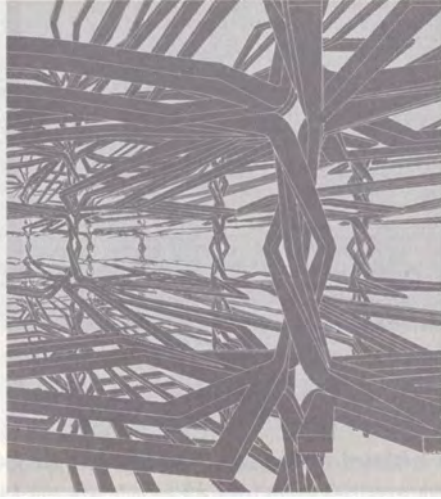
Görsel 72 Konrad Wachsmann, standart metal elemanlarla strüktür tasarımı (Konrad Wachsmann, Wendepunkt im Bauen , Krausskopf-Verlag, Wiesbaden, 1959, s. 201).
