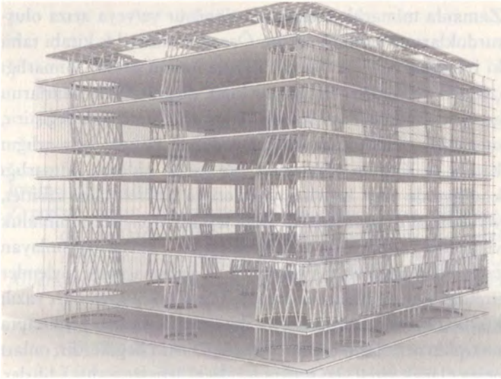
Görsel 86 Mühendislik-mimarlık bütünleşmesinin örnek tasarımlarından biri: Sendai Medyateği. 3d sitem görselleştirmesi (2001), mimar: Toyo Ito, mühendis: Mutsuro Sasaki.
