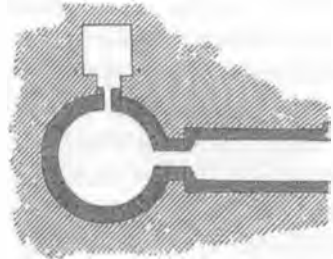
Mykenai kalesinin altındaki “Atreus’un Hazine Odası”nın kesiti ve planı.
