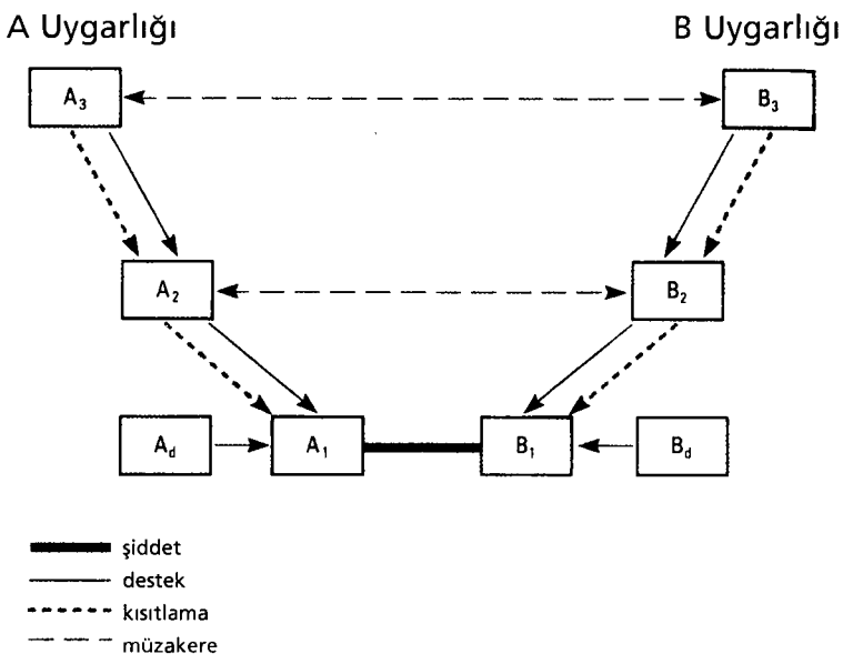
ŞEKİL 11.1 KARMAŞIK BİR FAY HATTI SAVAŞININ YAPISI
