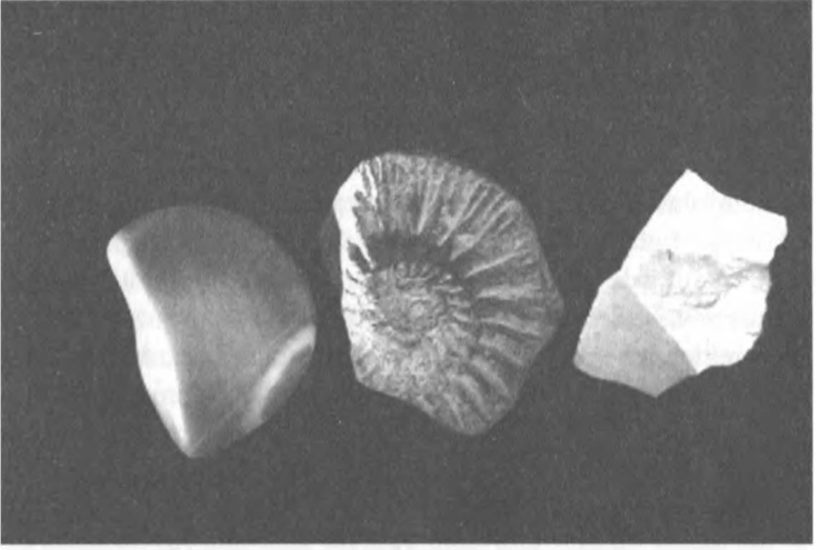
Resim 2: Üç sisteme örnekler: Sistem 1, kıyıda dalgalarla şekillenmiş doğal bir çakıltası (solda); Sistem 2, yumuşakça fosili; Sistem 3, çakmaktaşından üretilmiş bir aletin kırık parçası (sağda). (Fotoğraf yazara ait.)
