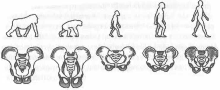
Şekil 8 - Kuyruksuz maymunlar ve insansıların pelvik morfolojisi, sol- dan sağa doğru: goril; şempanze; Australopithecus afarensis (Lucy); Ho- mo erectus (Gona); anatomik olarak modern insan.
