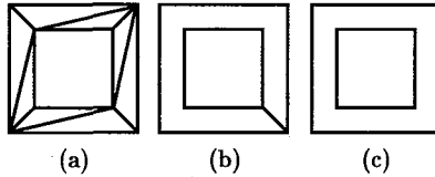
Şekil 14. Halka biçimli yüzün üç versiyonu: (a) Jonquières, (b) Matthiessen, (c) “eğitimsiz göz”.
