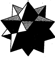
Şekil 7. Kepler'in yıldız-çokyüzlüsü; aynı beşgen yüzdeki üçgenler aynı biçimde taranmıştır.
