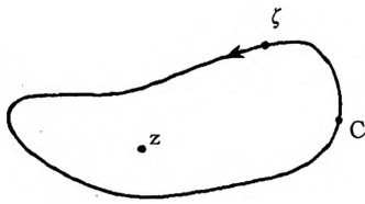
Şekil 18. Cauchy İntegral Formülü.
