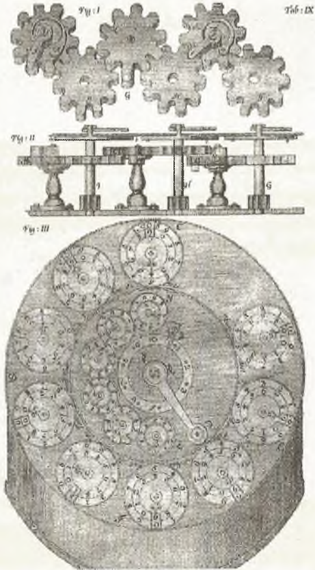
ŞEKİL 121. Jakob Leupold'un hesap makinesi (J. Leupold, Theatrum machinarum , 1727). 120
