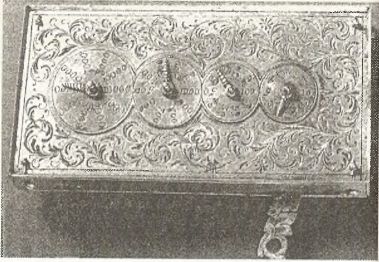
ŞEKİL 41. Adım sayacı (adımölçer, podometre < Yun. “ podion ”: adım + “ metron ”: ölçü) (1700 yılı dolayısı): Bu sayaç, yaya yürüyen bir insanın yanında taşınmakta ve sayaç kolu, bir ip ile ayağa bağlanmakta olup her iki adımda bir allayarak çift-adımları saymaktadır. Aletin üzerindeki göstergeler, 11 bin çift-adımın ölçümünü kapsamaktadır. 75
