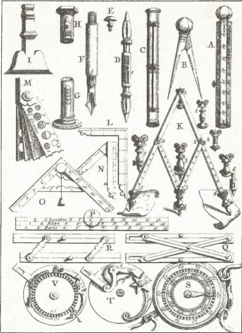
ŞEKİL 60. Nicolas Bion'un Traité de la construction et des principaux usages des instruments de mathématique (Den Haag, 1723; birinci baskısı Paris, 1709) adlı eserinden başka bir sayfada çeşitli ölçüm ve çizim aletleri: (A) ve (B) Çeşitli ölçeklere göre hegzagonal yapıda bölmeleyici (taksimatlayıcı); (C) ve (D) İki uçlu tebeşir tutacağı; (E), (F) ve (G) Erken bir dolmakalem tipinden görüntüler; (I) Bion'un kâğıt kuskacı; (K) Basit pantograf; (L), (N) ve (O) Çeşitli kuadrantlar (sonuncusu kurşun bir ağırlık asılarak düzcek olarak da kullanılabilmektedir); (P) Londra, Paris ve Rheinland için karşılaştırmalı üç dereceleme ölçeği ile birlikte ölçek cetveli; (Q) Makas bağlantılı paralel cetveli; (R) Köşegen bağlantılı paralel cetveli; (S) Podometre (admölçer); (T) ve (V) Ölçü tekerleri ( Science Museum Library , Londra). 84
