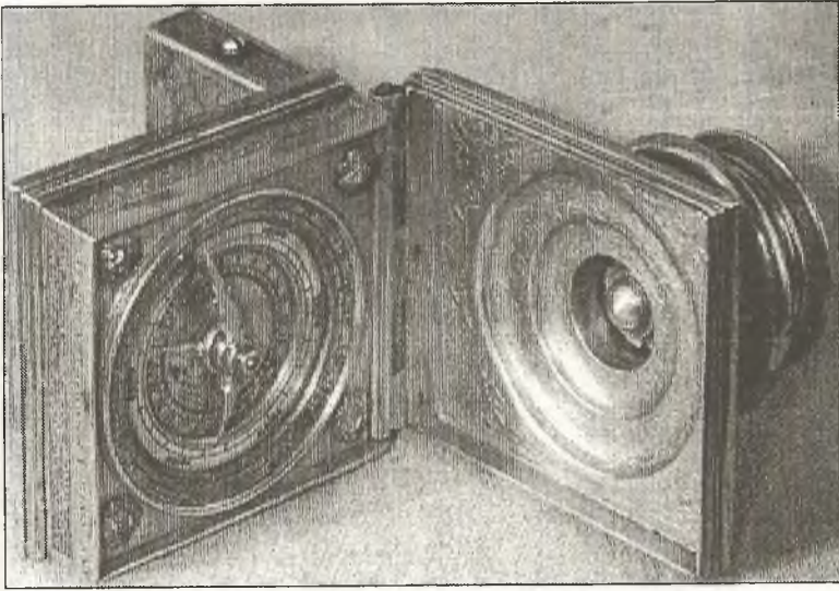
ŞEKİL 40. Thomas Rückert (~1532-1606) tarafından 1581'den sonra Augsburg'da yapılan bir adım sayacı. Pirinç üzeri altın kaplama; iki adet gümüş rakam kadranı bulunmakta; 6,8 x 6,2 cm; yükseklik 9 cm. Bu sayaç kemere takılırken kulp kısmı bir şeritle bacağına bağlanır ve her çift-adımda bir rakam atlar (Staatliche Museen Kassel, Museum für Astronomie und Technikgeschichte). 17
