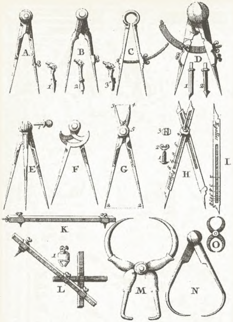
ŞEKİL 59. Nicolas Bion'un Traité de la construction et des principaux usages des instruments de mathématique (Den Haag, 1723; birinci baskısı Paris, 1709) adlı eserinden sekiz değişik pergel: (A) Sac pergeli, (B) Alman pergeli, (C) Kanatlı bölme pergeli, (D) Metal çizmeye yarayan kanatlı pergeli, (E) Uç ayaklı pergel, (F) Deniz haritası pergeli, (G) Sabit oranlı pergel, (K) Büyük daire çizmek için sürgülü pergel, (L) Eliptik pergel, (M) Küresel pergel, (N) Silindirik pergel, (O) Eşit ya da simetrik küresel pergel. Böyle aletlerin yer aldığı koleksiyonlar, kullanımdan çok, o dönemde zenginler için bir statü simgesi olarak derleniyordu (Science Museum Library, Londra). 84
