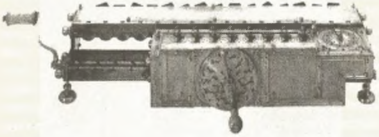
ŞEKİL 120. Gottfried Wilhelm Leibniz'in dört işlem yapan hesap makinesinin 1693 sonrası yapılan kopyası. 17
